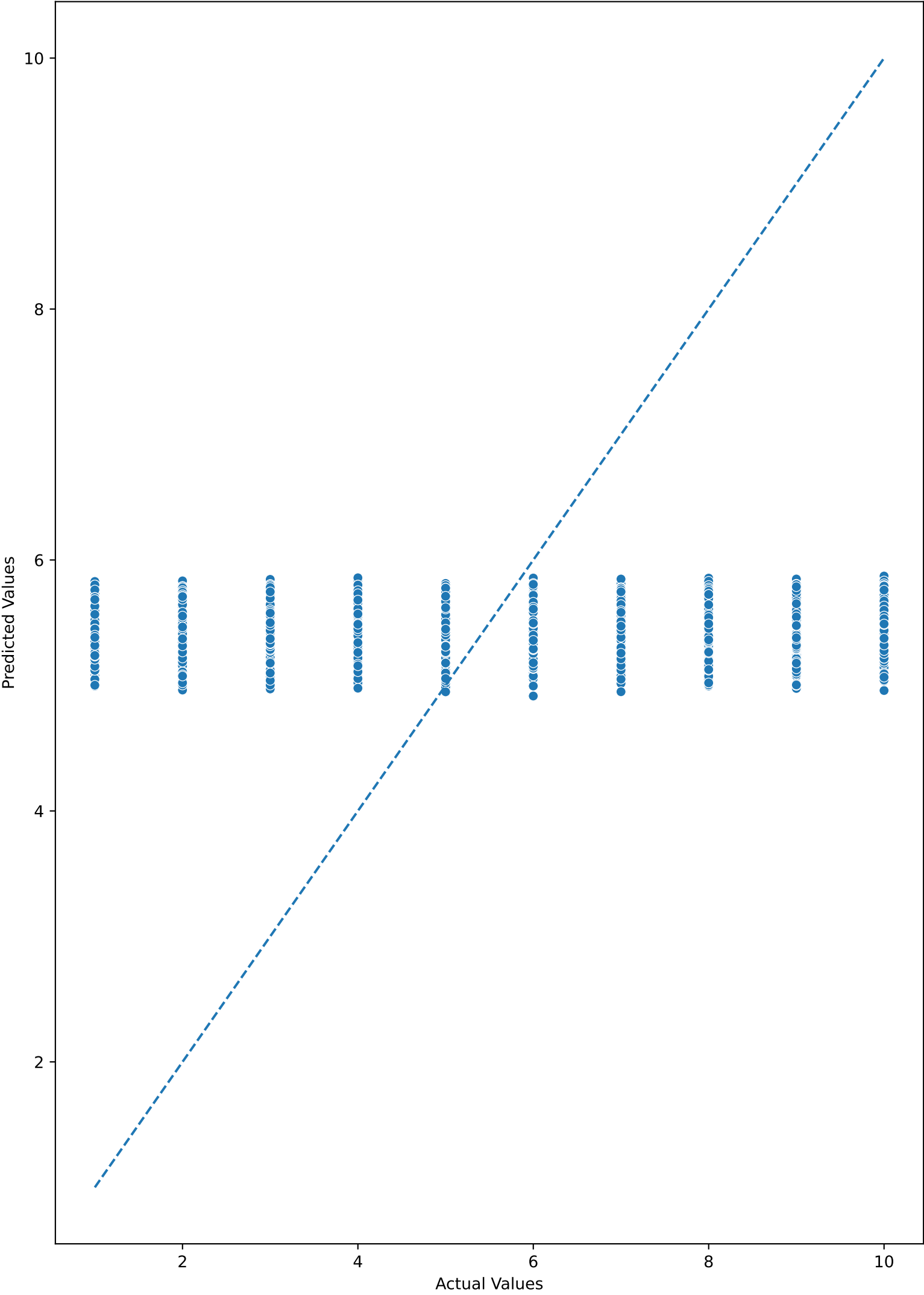
Actual vs Predicted - Ridge Regression
