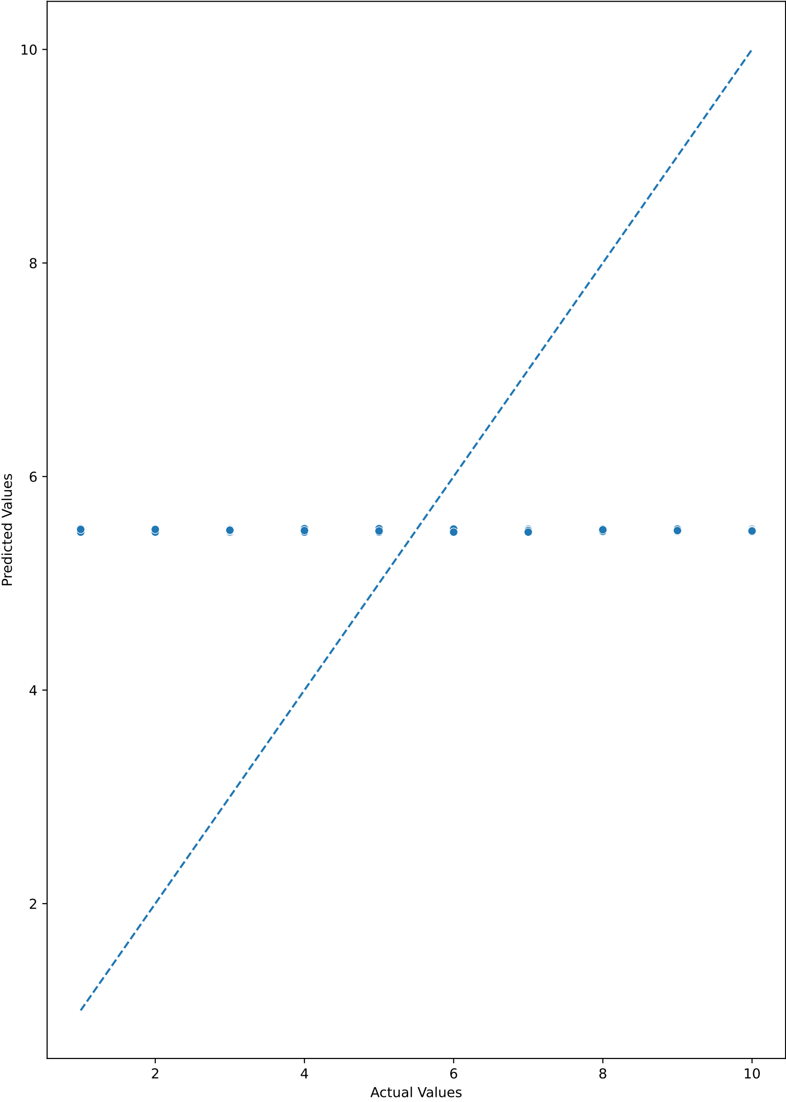
Actual vs Predicted - Lasso Regression
