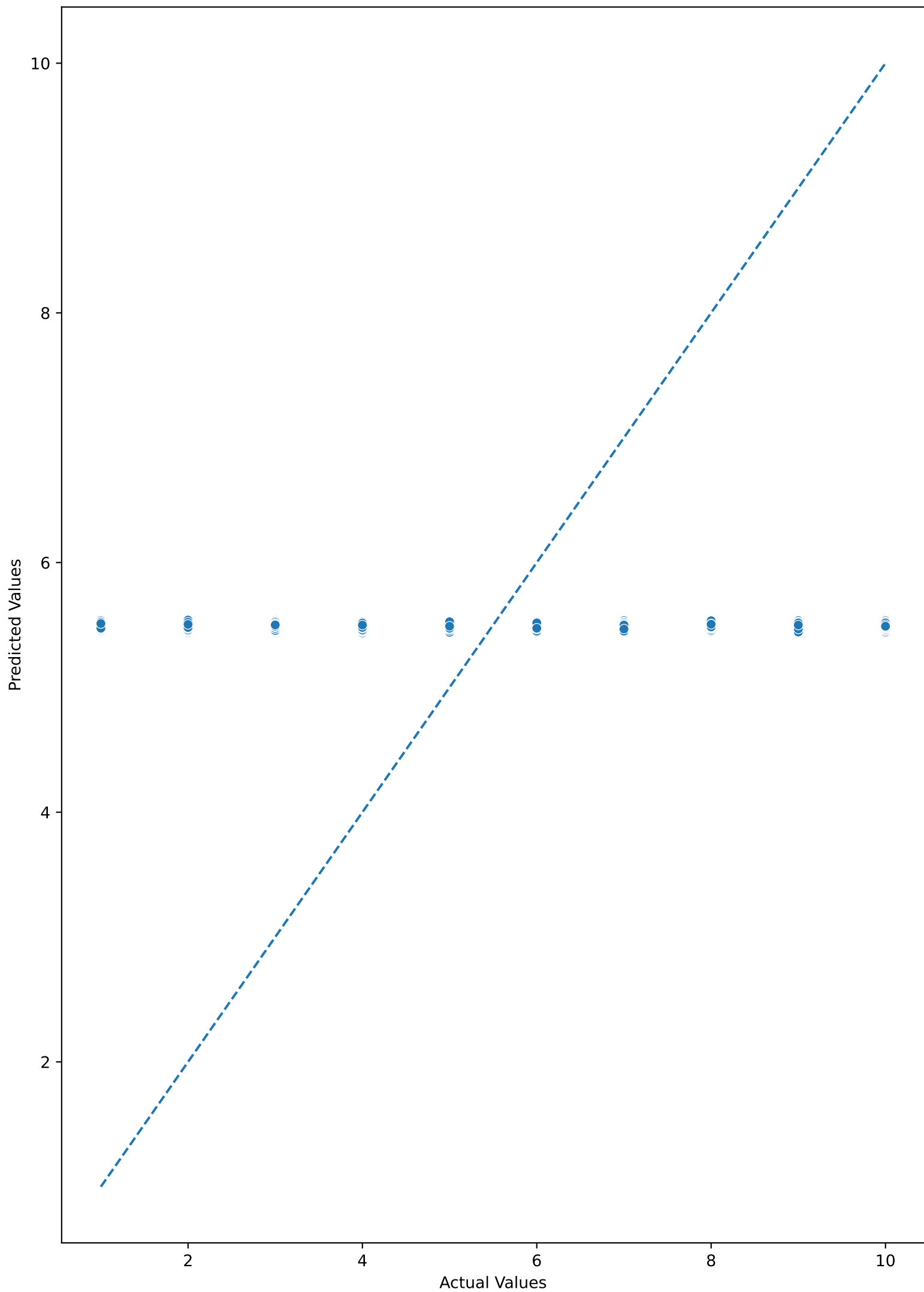
Actual vs Predicted - Elastic Net
