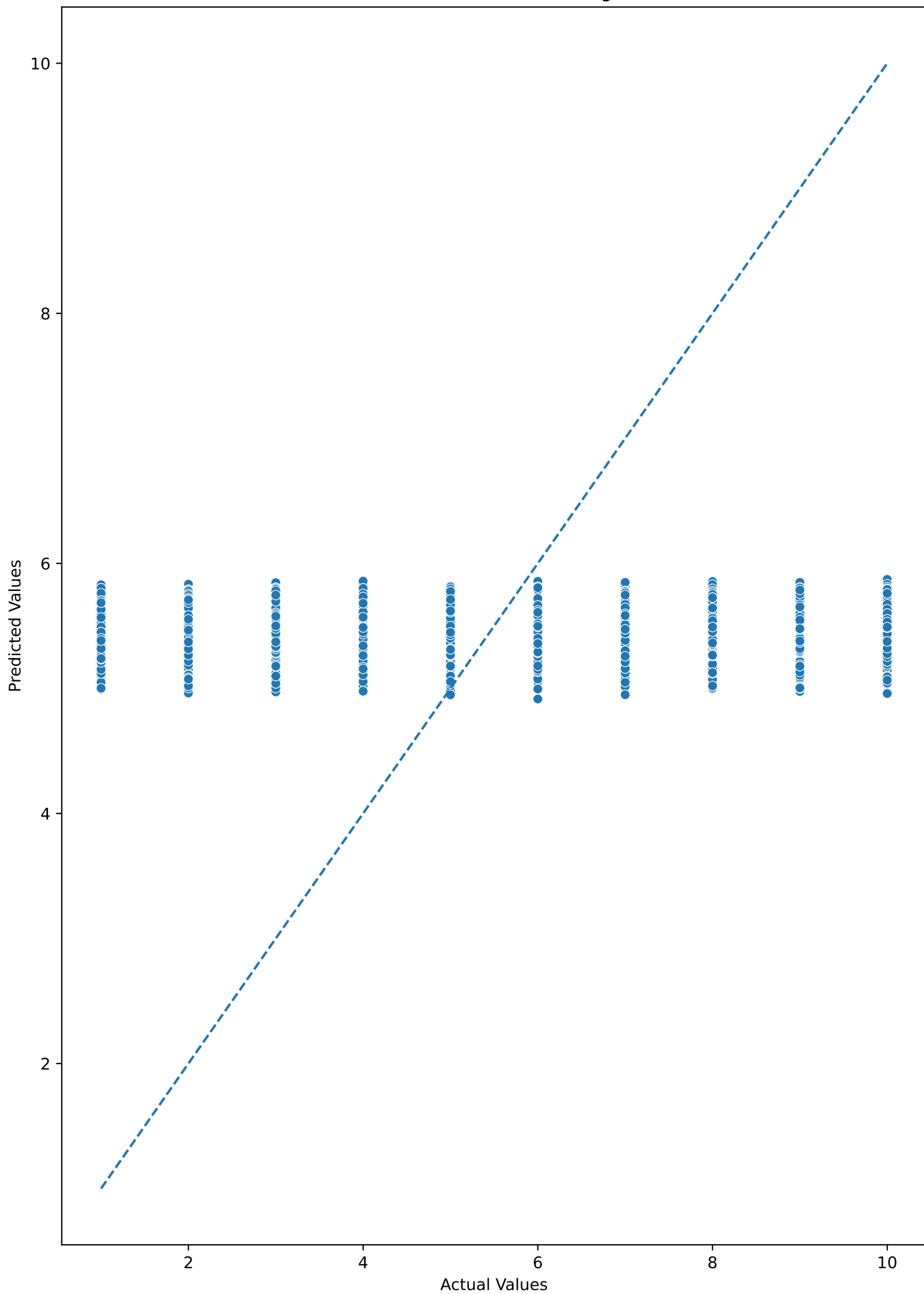
Actual vs Predicted - Linear Regression
