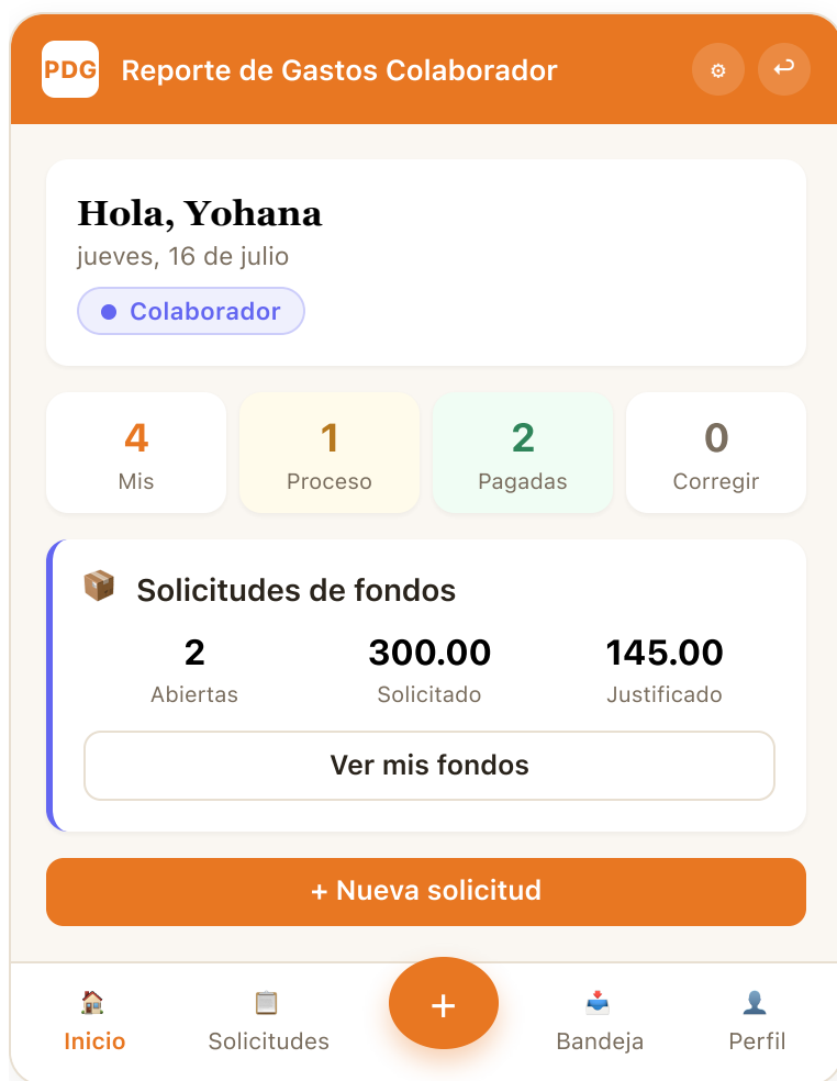
Fig. 5.1 – Home del colaborador con widget de fondos y navegación inferior.
