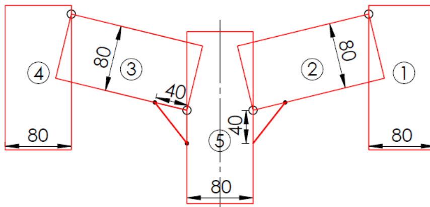
Estrutura 1.0 Pista
