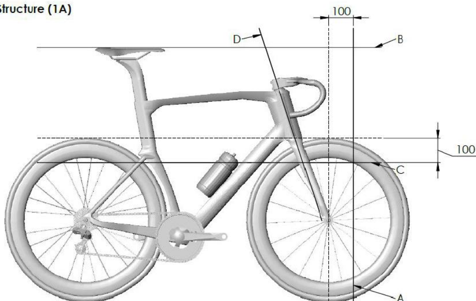
Structure (1A)
