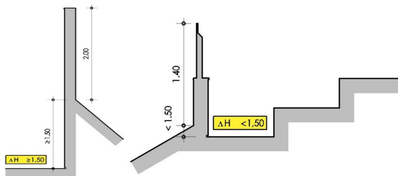
Diagrama demonstrativo da vedação exterior em diferentes alturas
