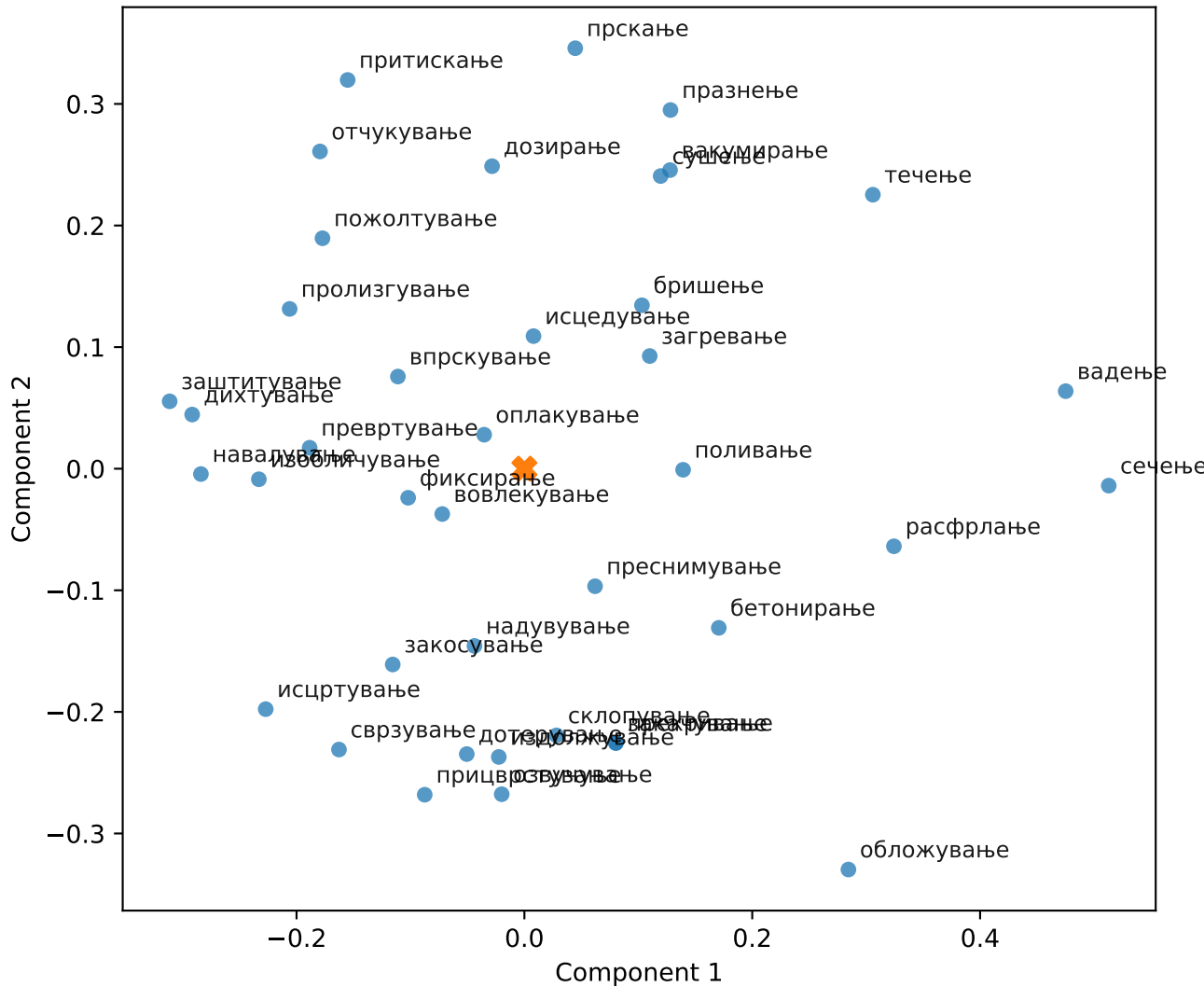
trained-mk_skipgram · parallel · K=200 · cid=103 · PCA
