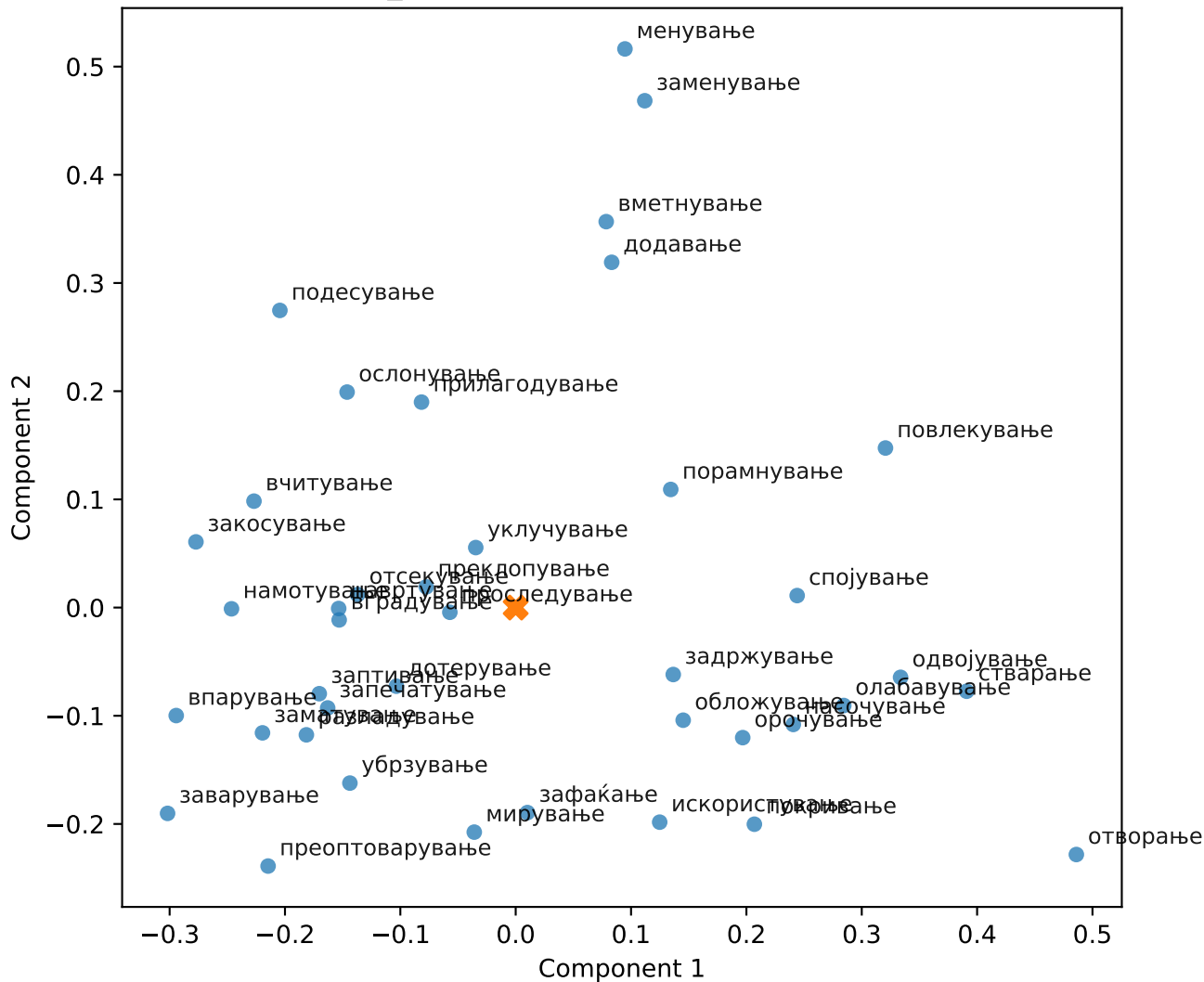
trained-mk_skipgram · serial · K=200 · cid=147 · PCA
