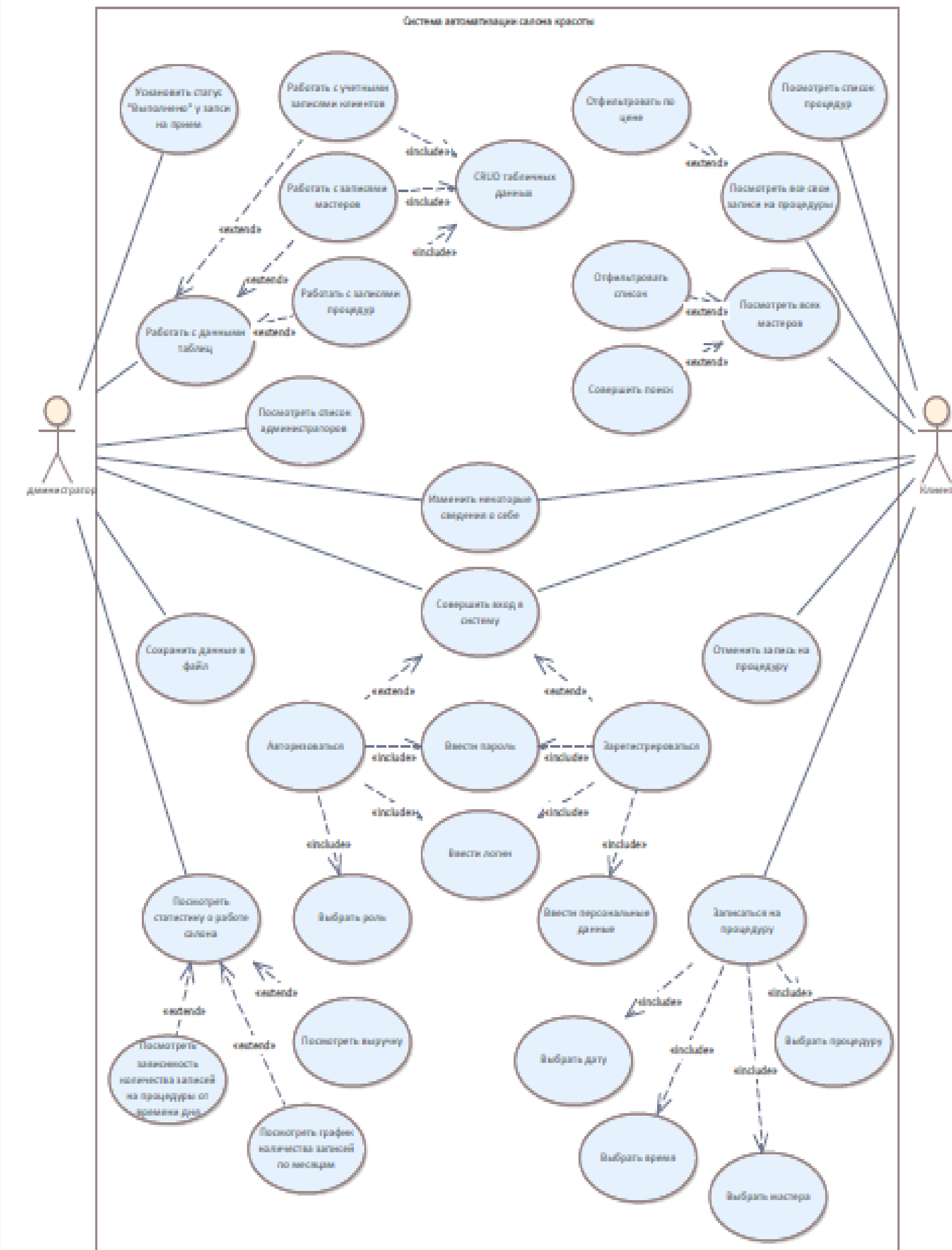
Диаграмма вариантов использования
