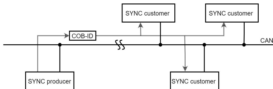
图 3-2 SYNC 架构
