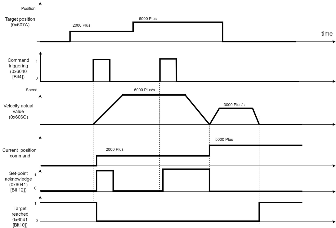
图 5-4 PP 模式非立即生效命令指令时序图
