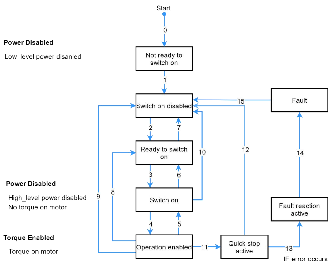
图 5-1 设备状态机
