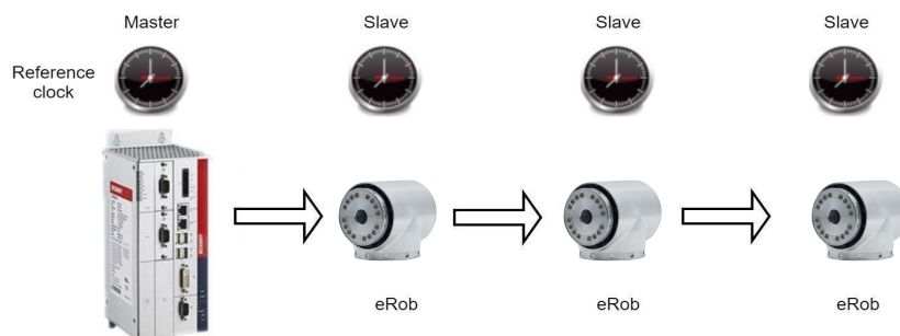
图 4-3 时钟同步架构
