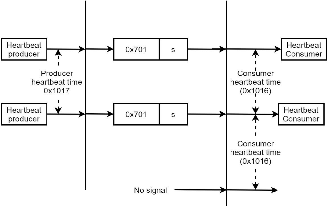
图 3-7 Heartbeat 模型
