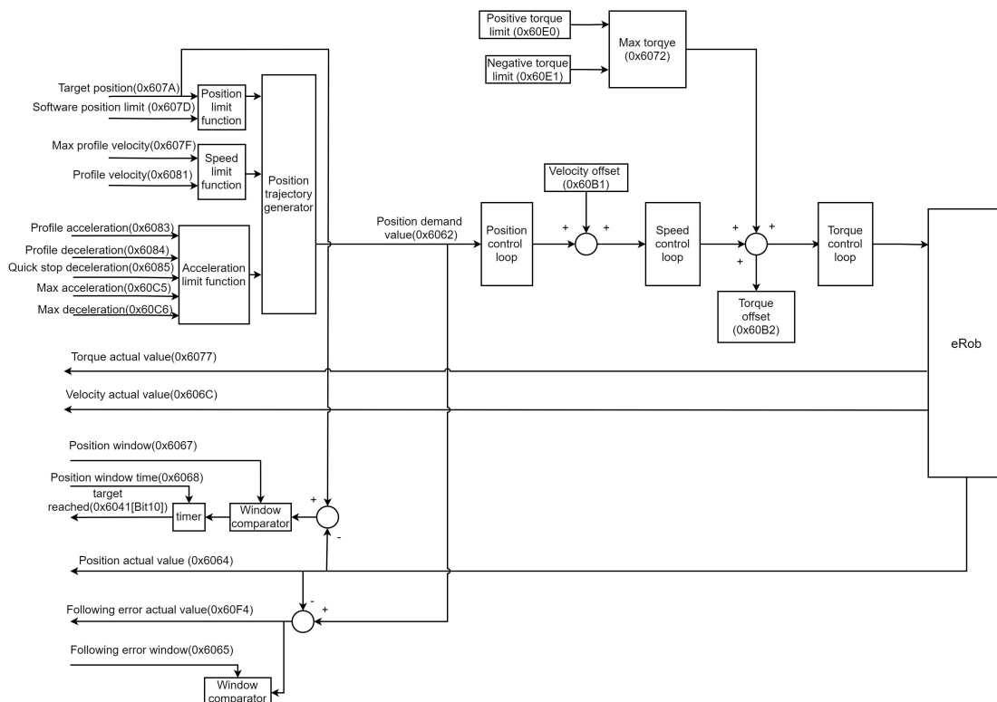
图 5-3 PP 模式的功能
