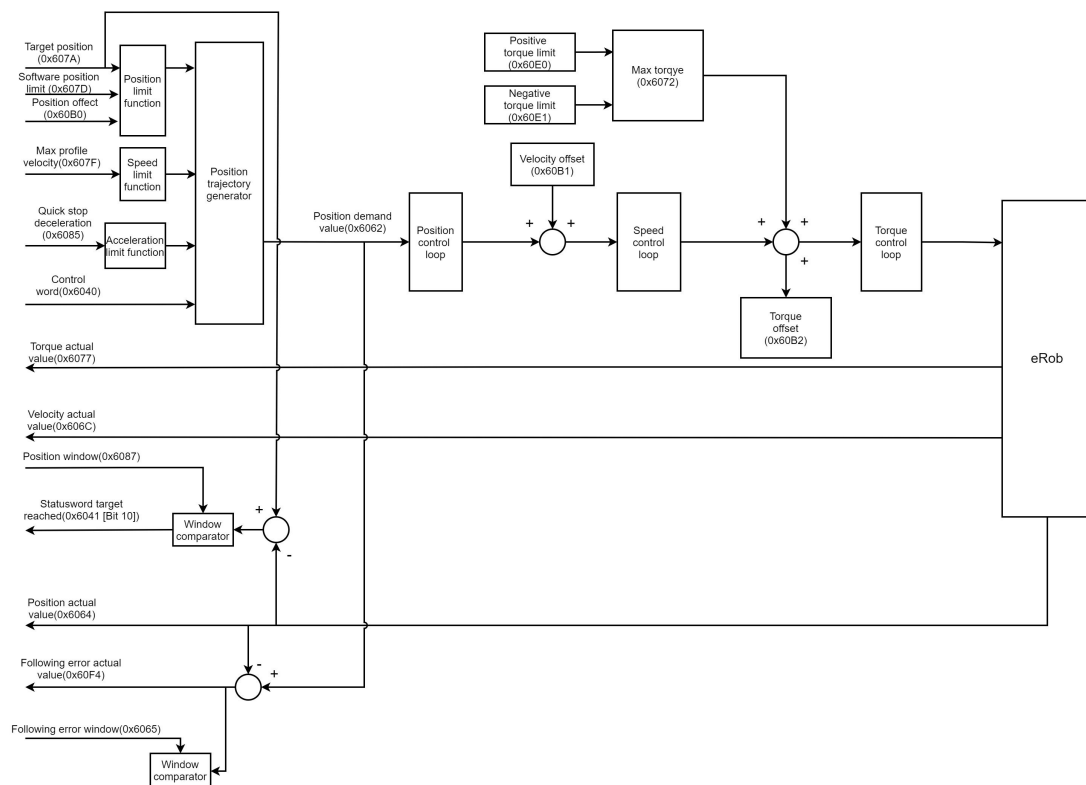
图 5-2 CSP 模式的功能
