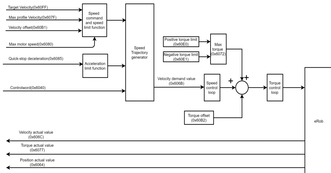
图 5.6 CSV 模式的功能
