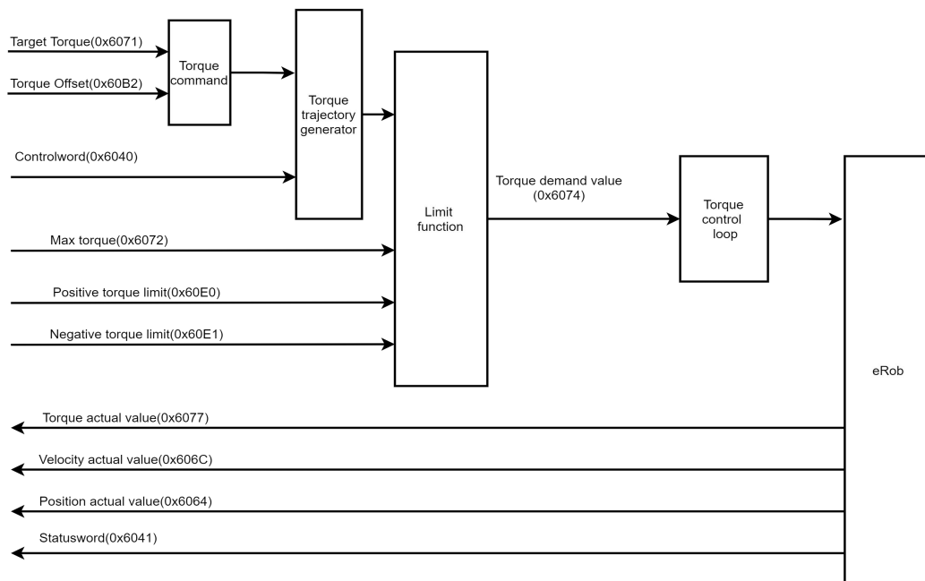
Figure 5-8 CST 模式的功能
