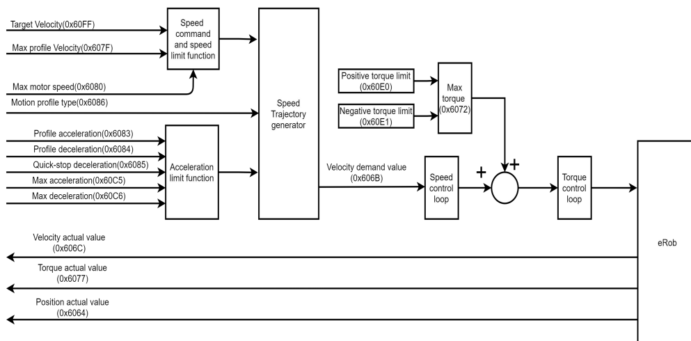
图 5.7 PV 模式的功能
