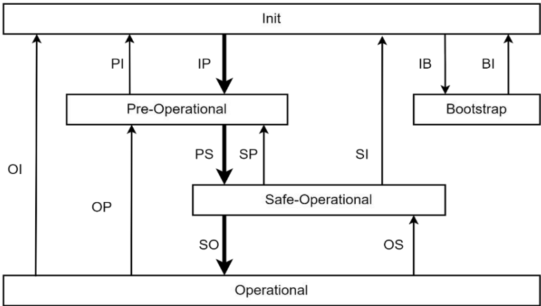
图 4-2 EtherCAT 状态机
