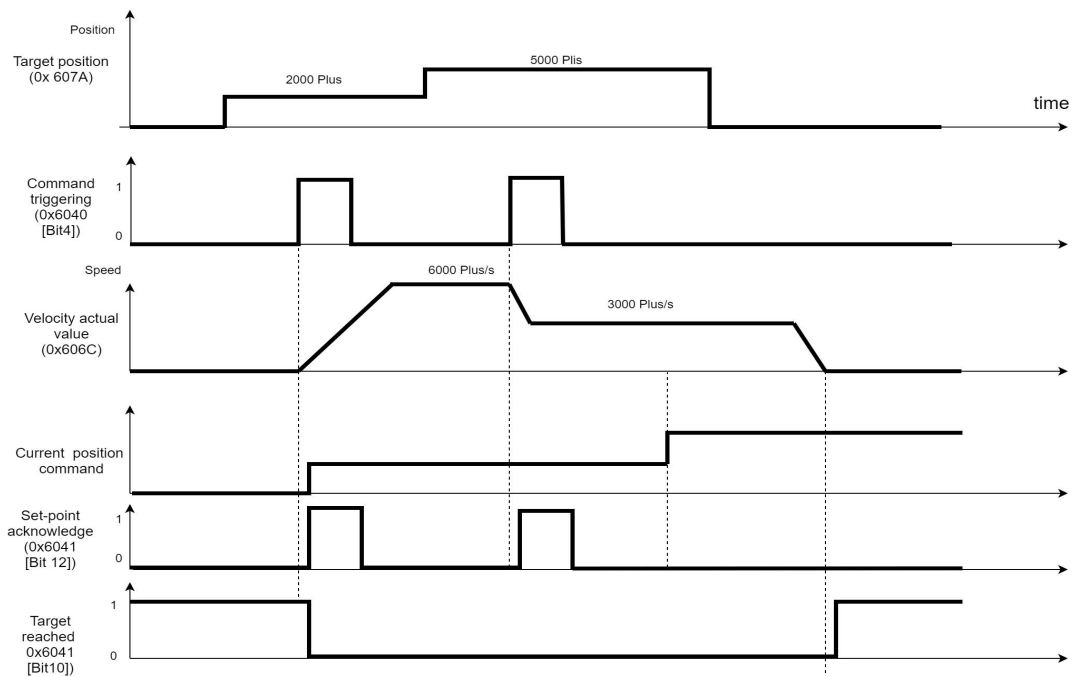
图 5.5 PP 模式立即生效指令时序图
