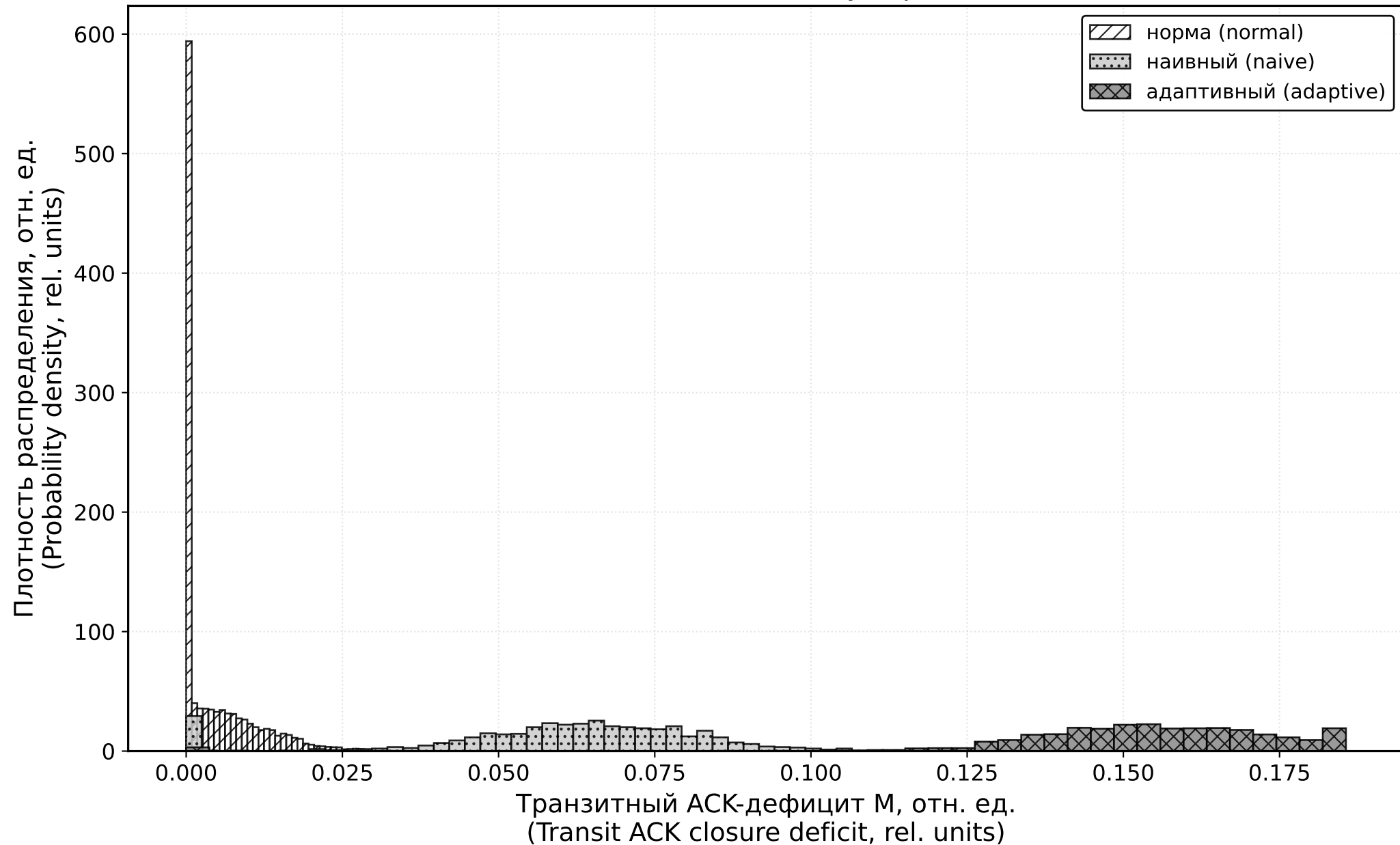
Рисунок 4 — Распределение АСК-инварианта: адаптивный противник смещён ВПРАВО (неустраняемый след) (ACK invariant distribution by sophistication)
