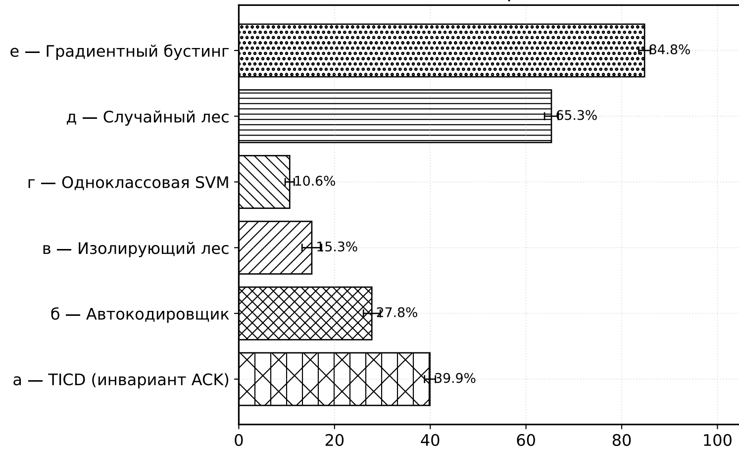
(г) Полнота компрометации, % (Compromise recall)
