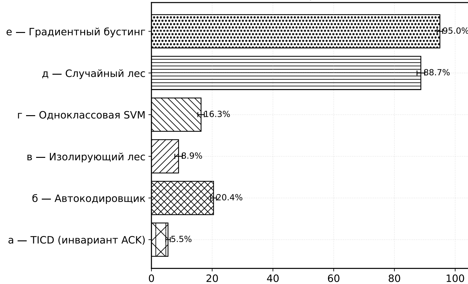
(а) Полнота при FPR=1%, % (Recall @1% FPR)
