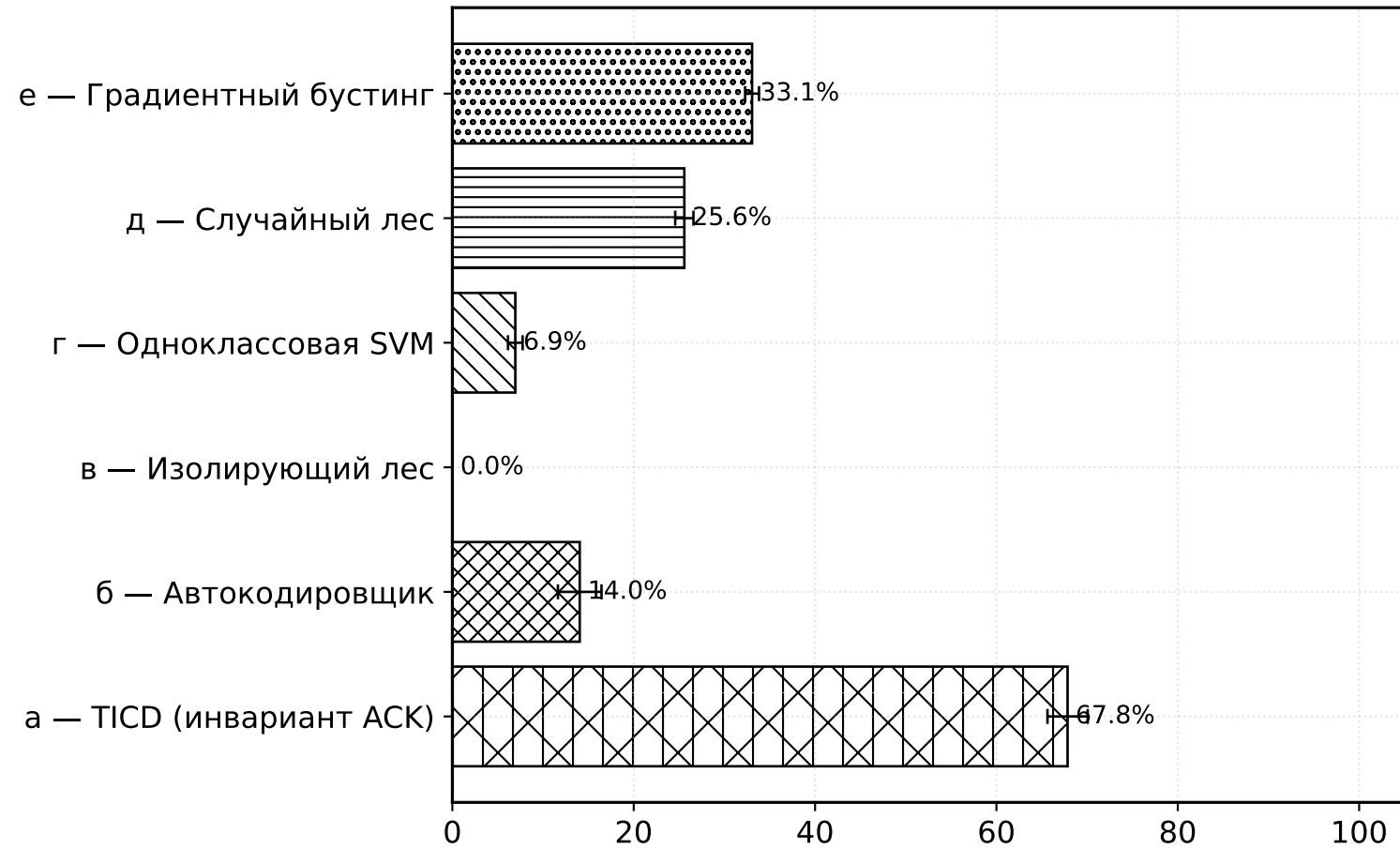
(б) Полнота на адаптивном, % (Adaptive recall)
