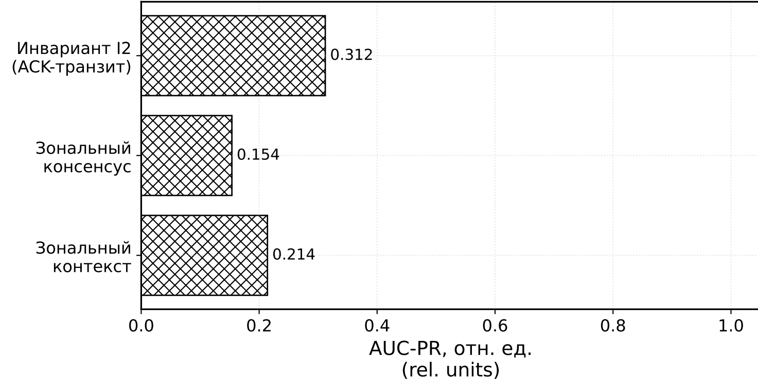
(б) AUC-PR
