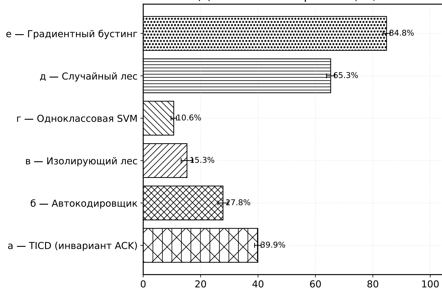
(г) Полнота компрометации, % (Compromise recall)
