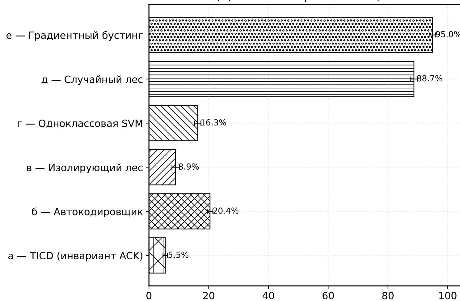
(а) Полнота при FPR=1%, % (Recall @1% FPR)
