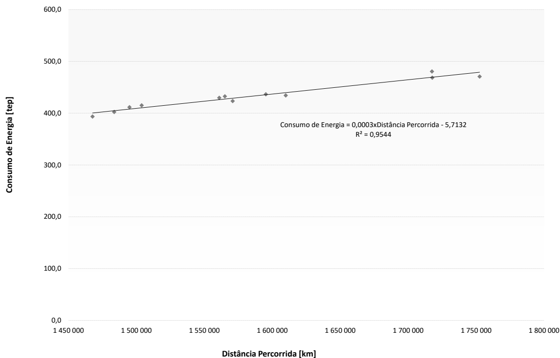
Gráfico 5 - Consumo de energia vs distância percorrida - Veículos Mistos
