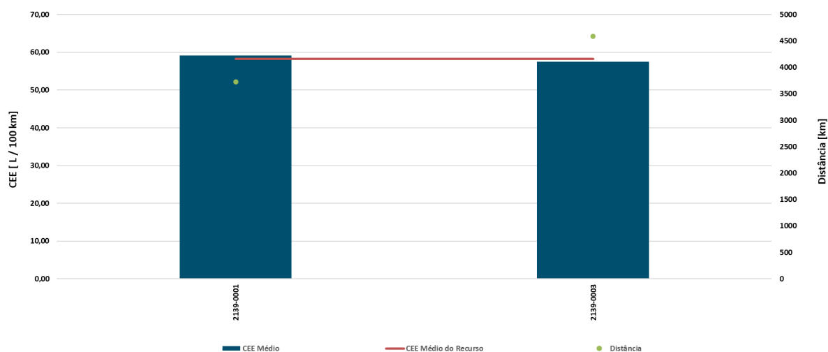
Gráfico 26 - Consumo específico médio e distância percorrida pelas viaturas RP.02.01.39
