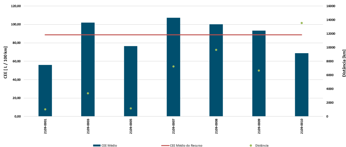
Gráfico 23 - Consumo específico médio e distância percorrida pelas viaturas RP.02.01.09
