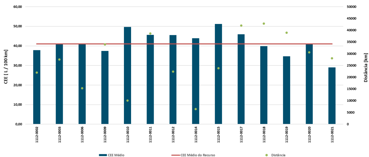
Gráfico 11 - Consumo específico médio e distância percorrida pelas viaturas RP.01.01.12
