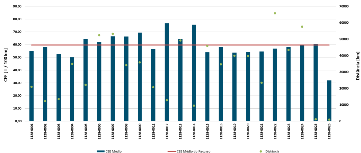
Gráfico 16 - Consumo específico médio e distância percorrida pelas viaturas RP.01.01.28
