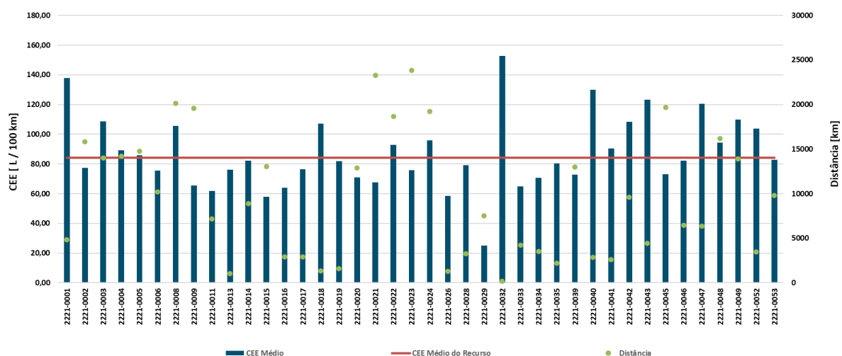
Gráfico 30 - Consumo específico médio e distância percorrida pelas viaturas RP.02.02.21
