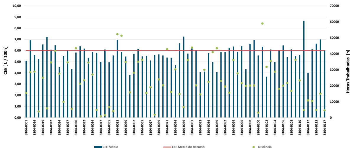
Gráfico 32 - Consumo específico médio e distância percorrida pelas viaturas RE.08.01.04
