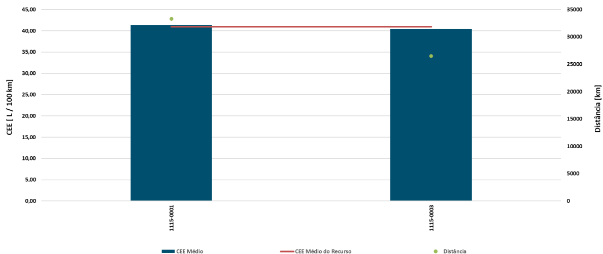
Gráfico 12 - Consumo específico médio e distância percorrida pelas viaturas RP.01.01.15
