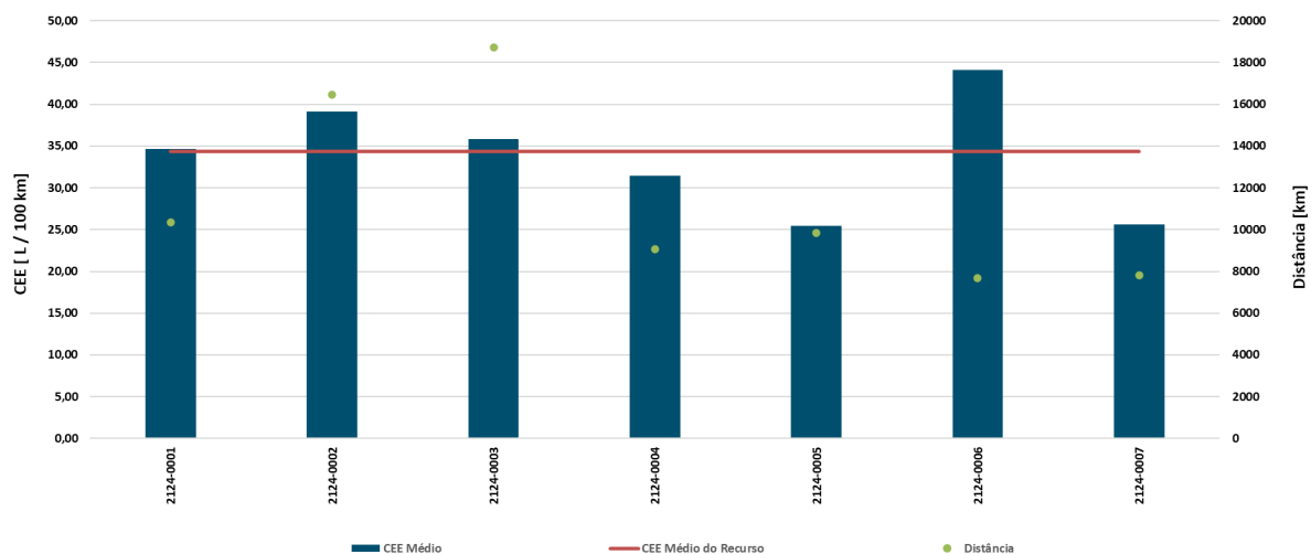
Gráfico 24 - Consumo específico médio e distância percorrida pelas viaturas RP.02.01.24
