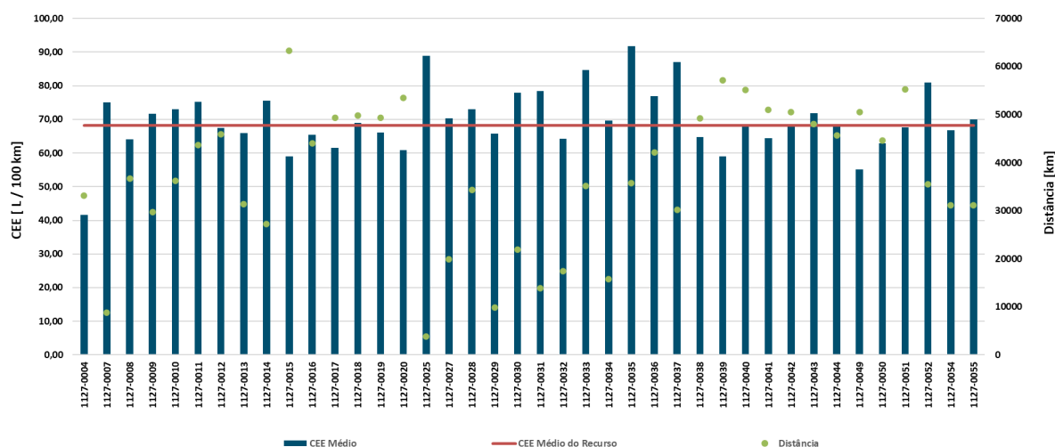
Gráfico 15 - Consumo específico médio e distância percorrida pelas viaturas RP.01.01.27
