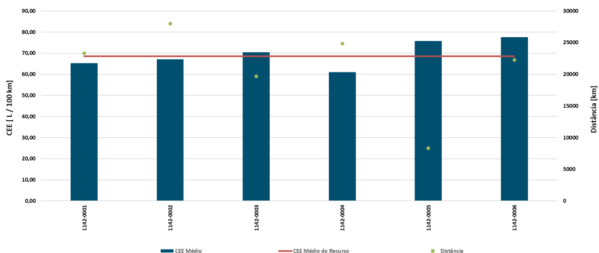
Gráfico 17 - Consumo específico médio e distância percorrida pelas viaturas RP.01.01.42
