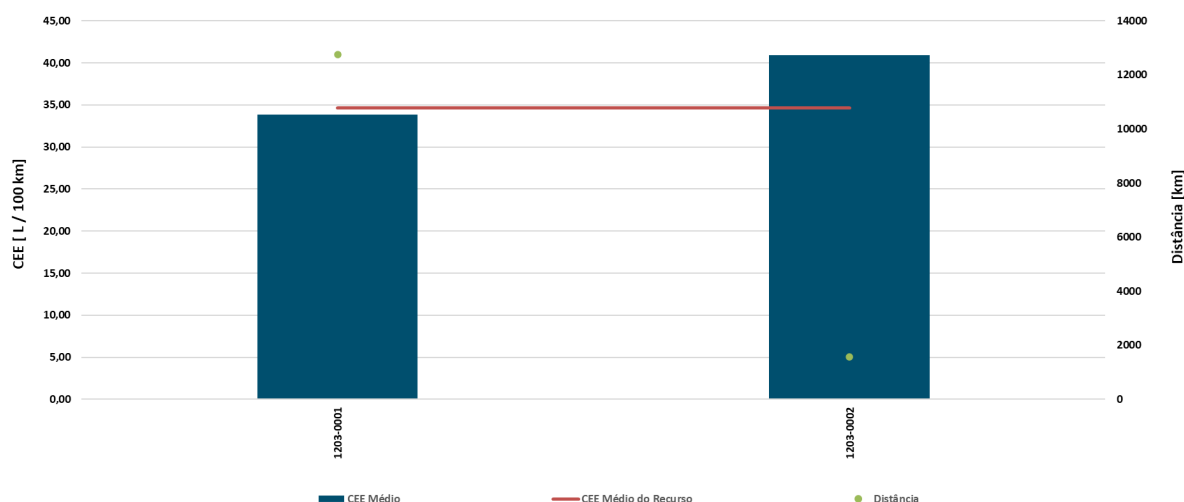
Gráfico 18 - Consumo específico médio e distância percorrida pelas viaturas RP.01.02.03
