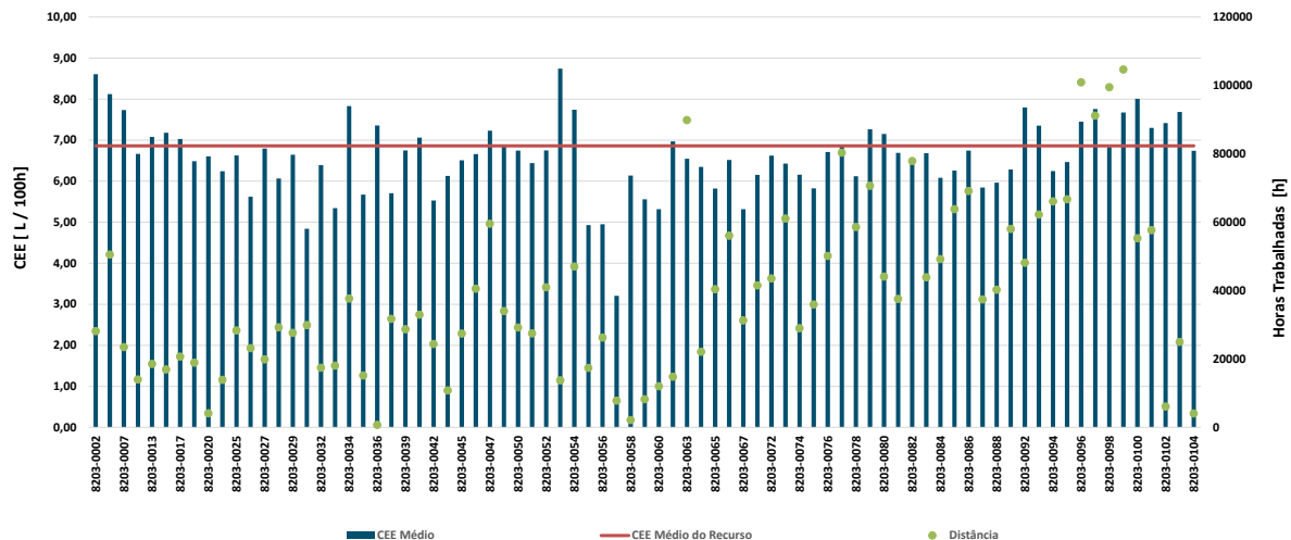
Gráfico 33 - Consumo específico médio e distância percorrida pelas viaturas RE.08.02.03
