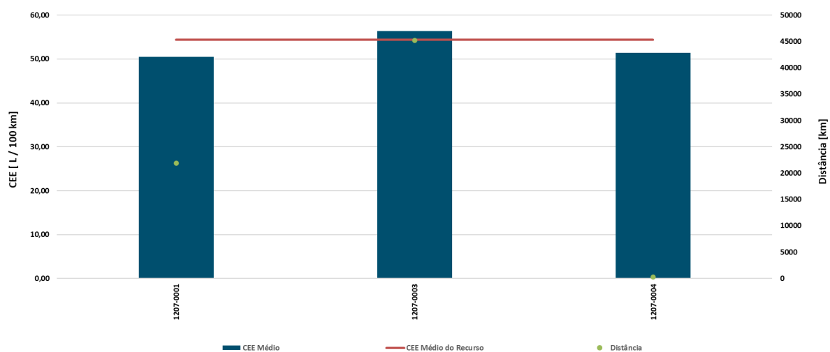
Gráfico 20 - Consumo específico médio e distância percorrida pelas viaturas RP.01.02.07
