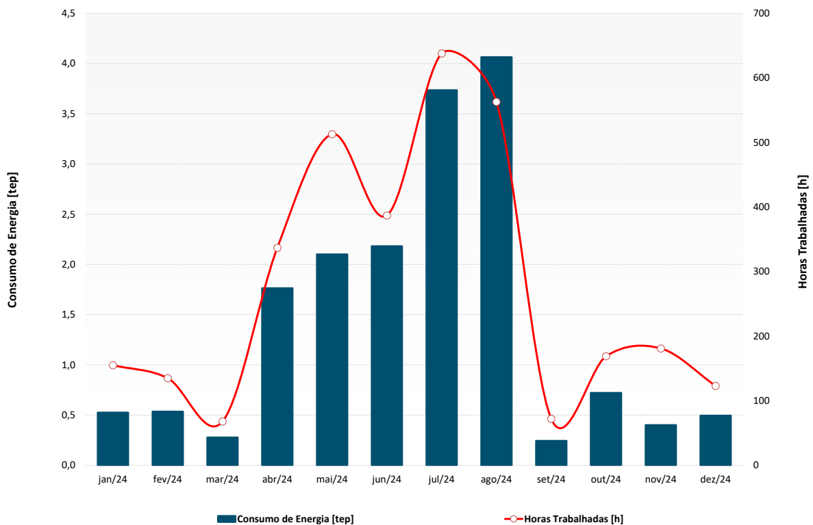
Gráfico 6 - Evolução do consumo de energia e das horas trabalhadas - Veículos Especiais
