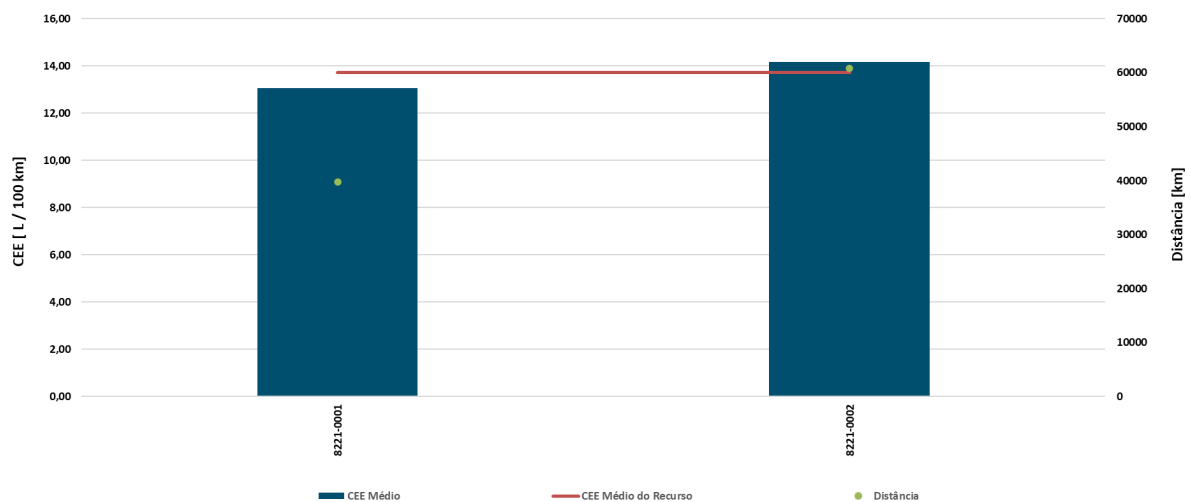
Gráfico 38 - Consumo específico médio e distância percorrida pelas viaturas RE.08.02.21
