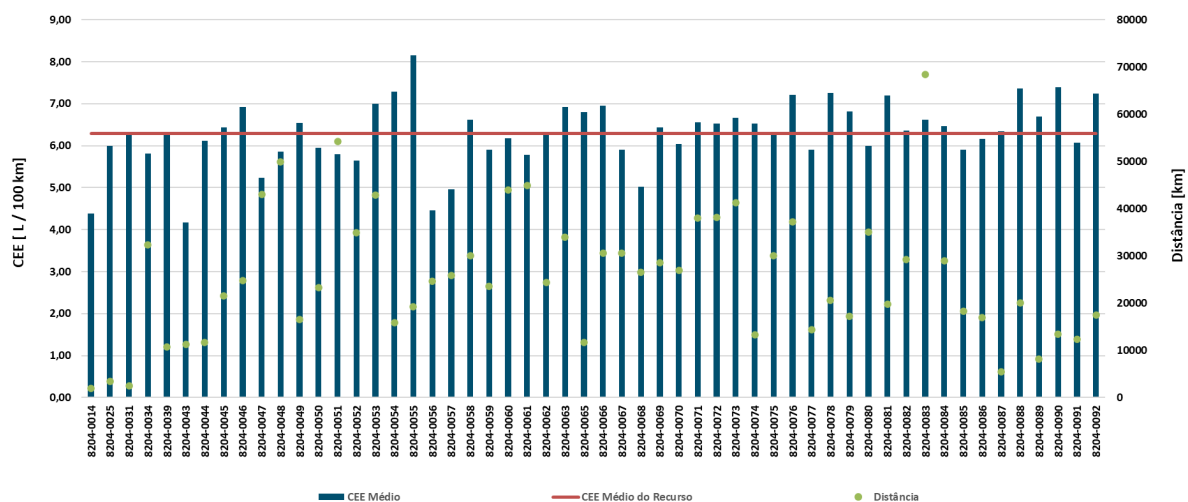
Gráfico 34 - Consumo específico médio e distância percorrida pelas viaturas RE.08.02.04
