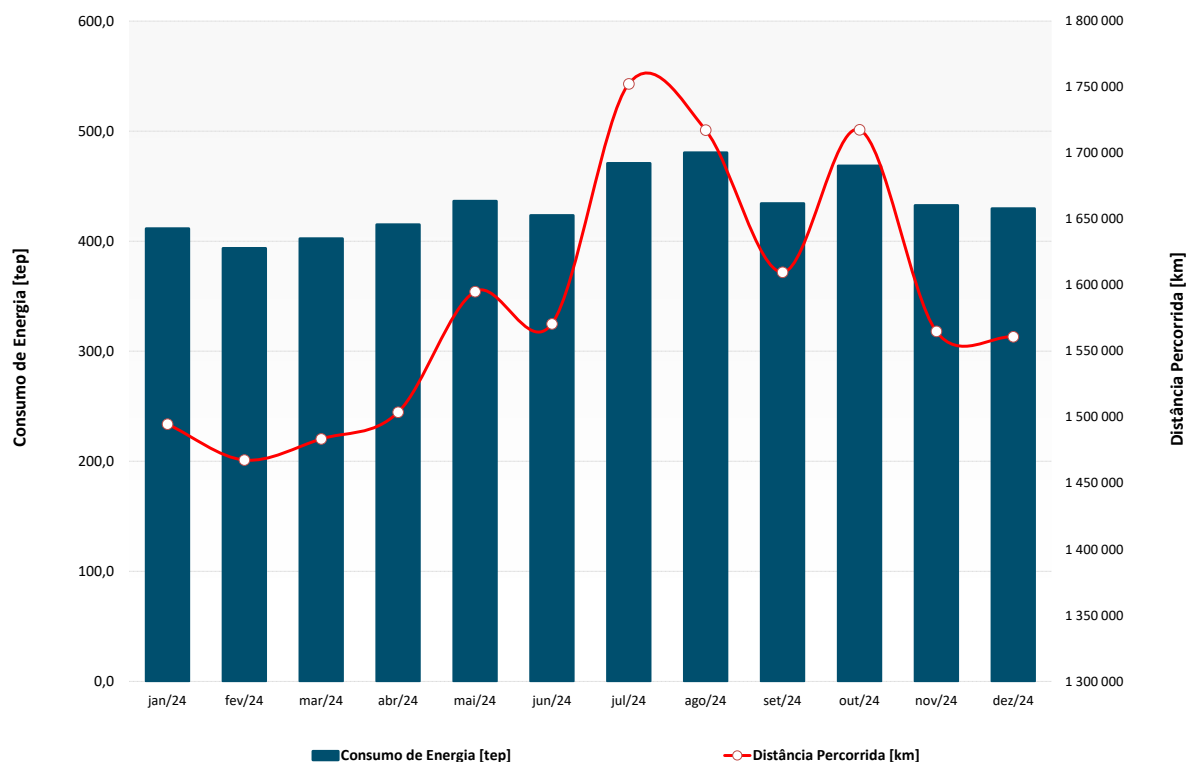
Gráfico 4 - Evolução do consumo de energia e da distância percorrida - Veículos Mistos
