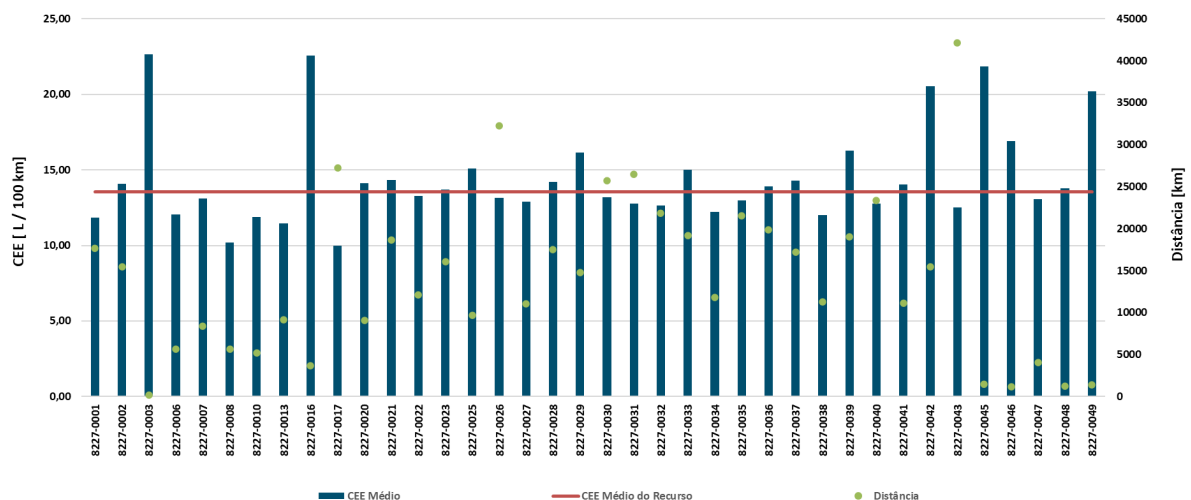
Gráfico 40 - Consumo específico médio e distância percorrida pelas viaturas RE.08.02.27
