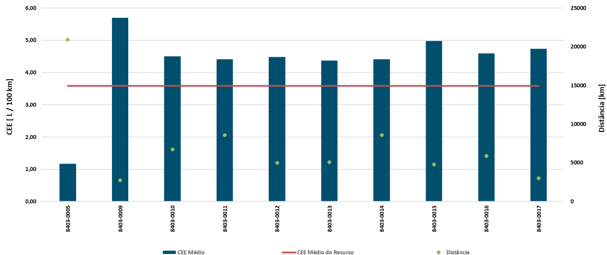
Gráfico 41 - Consumo específico médio e distância percorrida pelas viaturas RE.08.04.03
