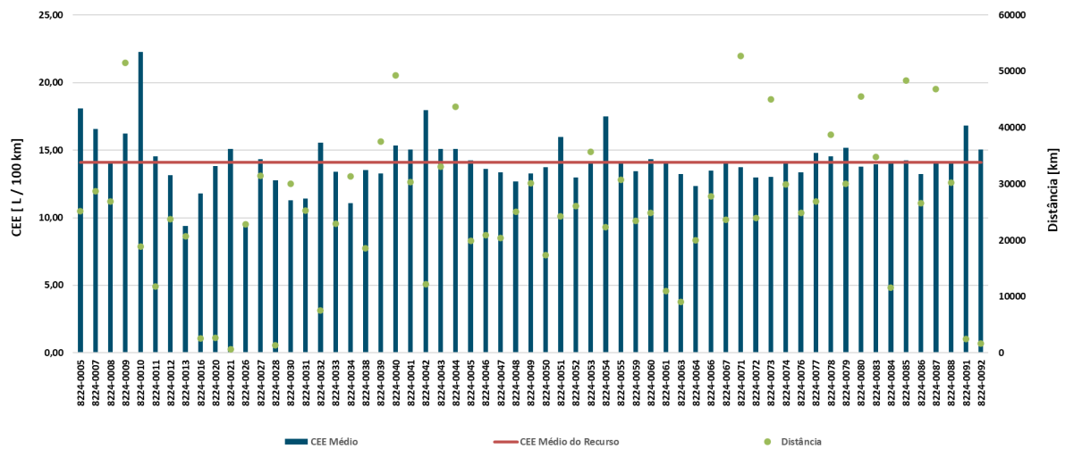
Gráfico 39 - Consumo específico médio e distância percorrida pelas viaturas RE.08.02.24
