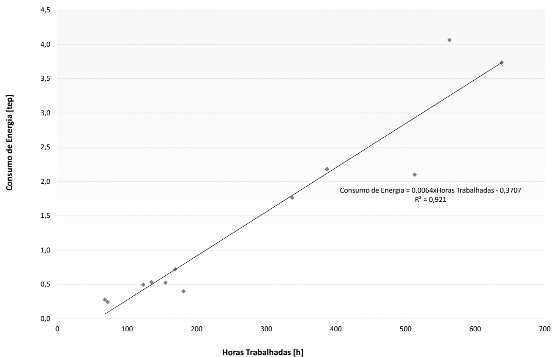
Gráfico 7 - Consumo de energia vs horas trabalhadas - Veículos Especiais
