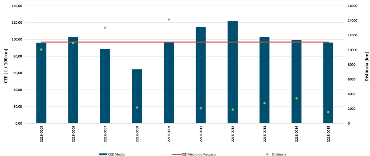
Gráfico 29 - Consumo específico médio e distância percorrida pelas viaturas RP.02.02.18
