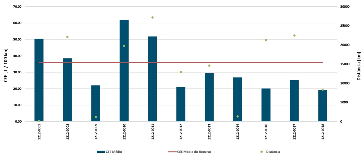
Gráfico 22 - Consumo específico médio e distância percorrida pelas viaturas RP.01.02.12
