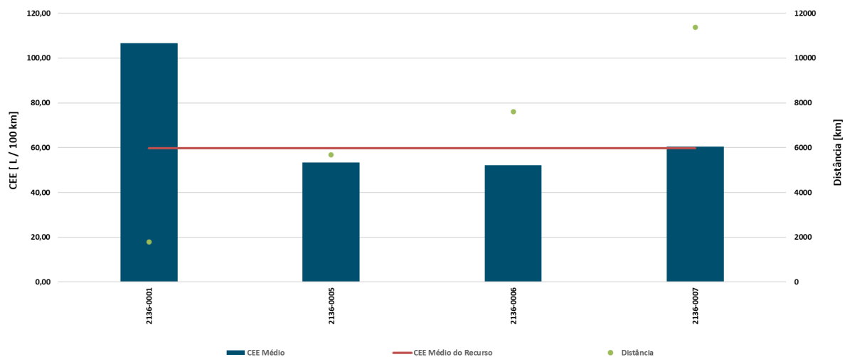
Gráfico 25 - Consumo específico médio e distância percorrida pelas viaturas RP.02.01.36
