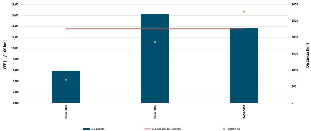
Gráfico 42 - Consumo específico médio e distância percorrida pelas viaturas RE.08.04.06
