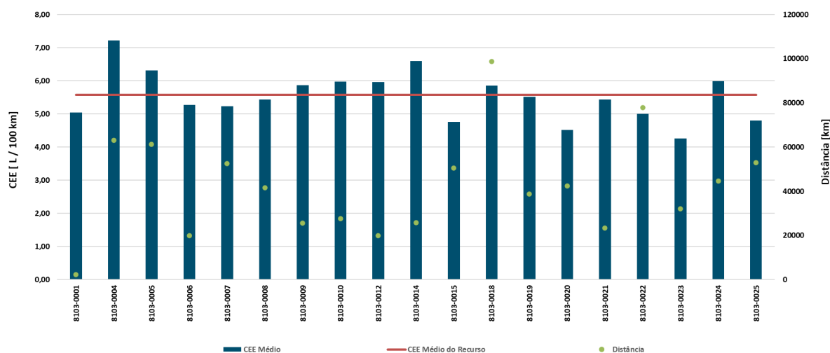
Gráfico 31 - Consumo específico médio e distância percorrida pelas viaturas RE.08.01.03
