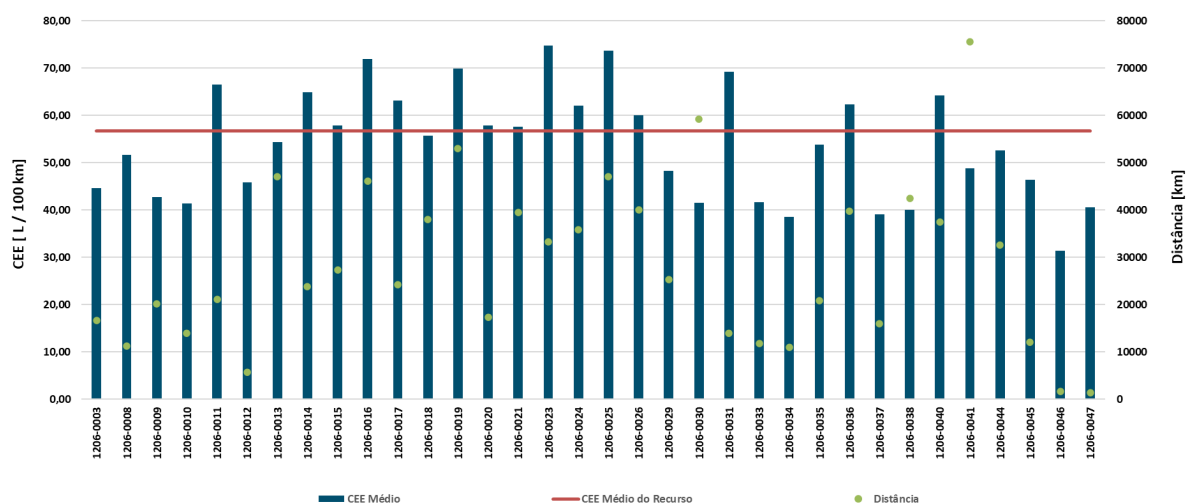
Gráfico 19 - Consumo específico médio e distância percorrida pelas viaturas RP.01.02.06
