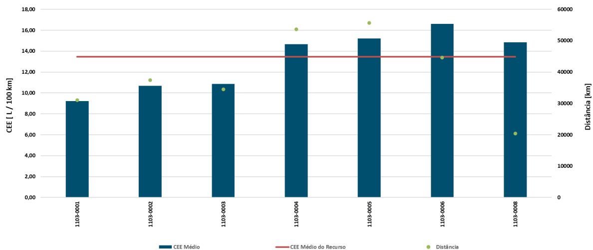
Gráfico 8 - Consumo específico médio e distância percorrida pelas viaturas RP.01.01.03
