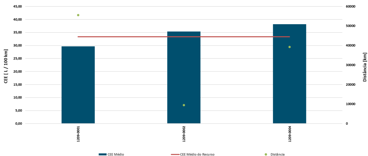
Gráfico 21 - Consumo específico médio e distância percorrida pelas viaturas RP.01.02.09
