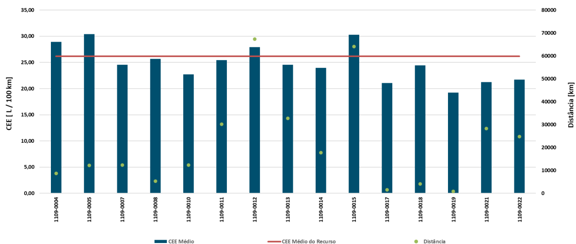
Gráfico 10 - Consumo específico médio e distância percorrida pelas viaturas RP.01.01.09
