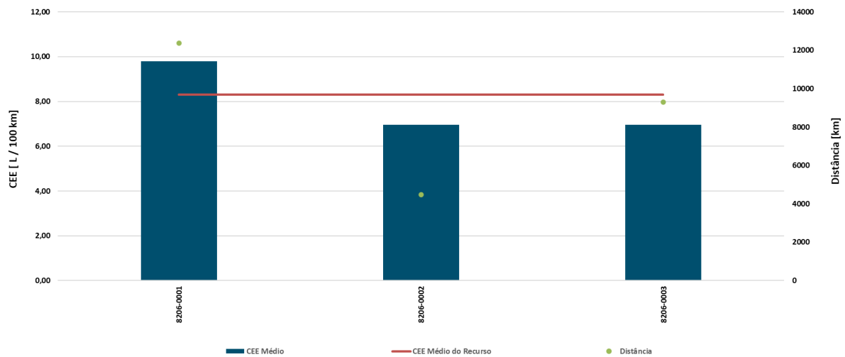
Gráfico 35 - Consumo específico médio e distância percorrida pelas viaturas RE.08.02.06
