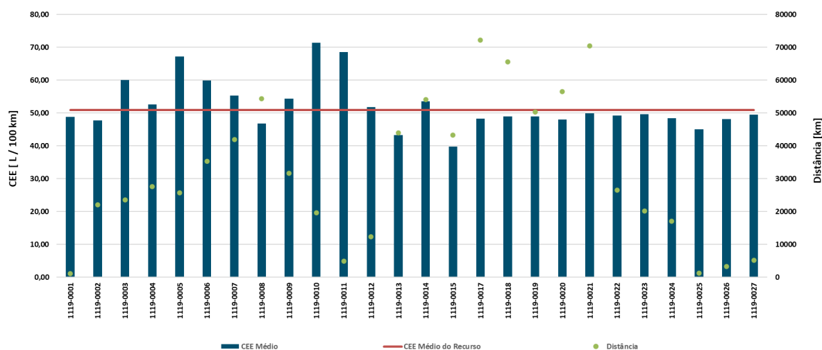
Gráfico 14 - Consumo específico médio e distância percorrida pelas viaturas RP.01.01.19
