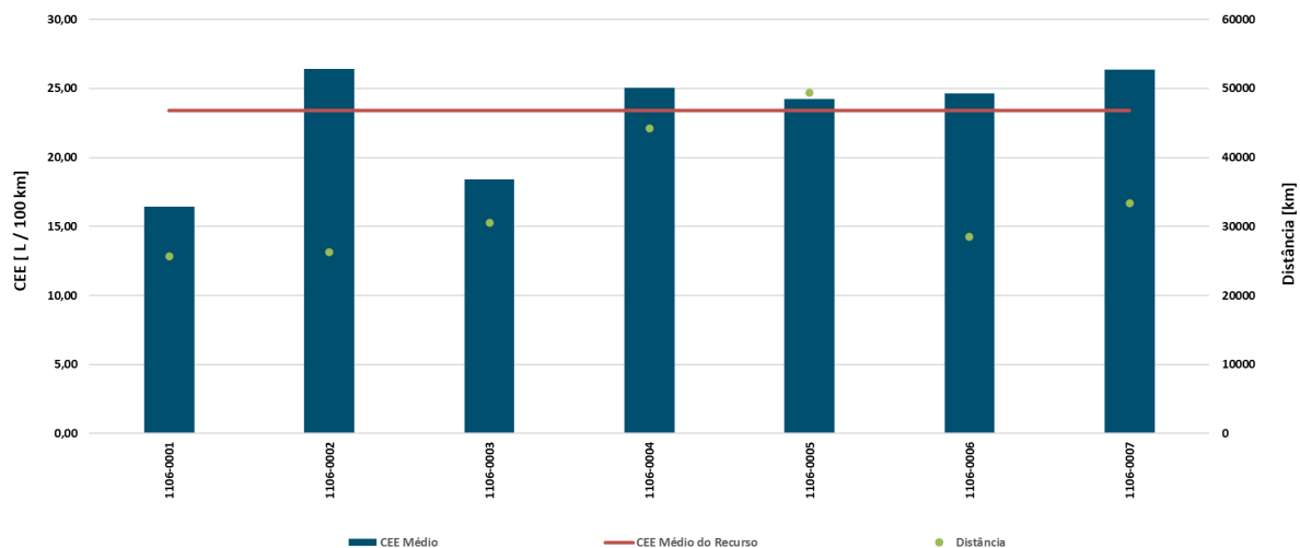
Gráfico 9 - Consumo específico médio e distância percorrida pelas viaturas RP.01.01.06
