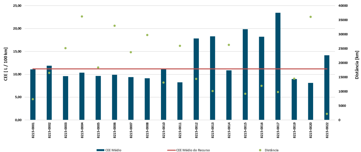
Gráfico 36 - Consumo específico médio e distância percorrida pelas viaturas RE.08.02.15
