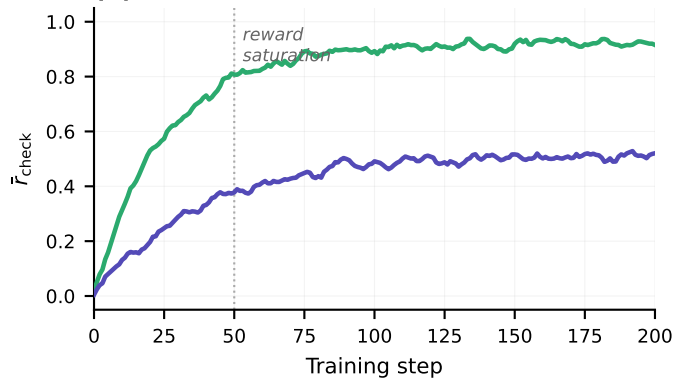
(d) Mean checker reward
