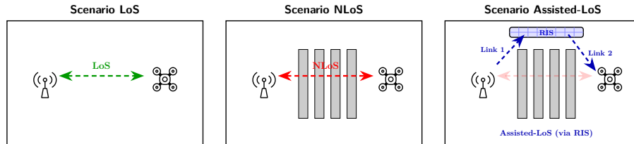
Figura 2: Confronto schematico tra condizione di visibilità diretta (LoS) e ostruzione totale (NLoS) in ambiente industriale magazzino.
