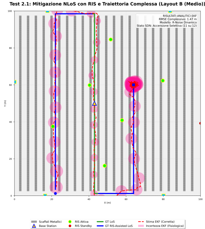
Figura 14: Test 2: Con la RIS attiva per A-LoS interviene il ripristino EKF metrico.
