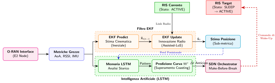
Figura 7: Diagramma di Flusso della Fusione Sensoriale Ibrida. Il sistema orchestra parallelamente l'elaborazione inerziale sub-metrica tramite Extended Kalman Filter (EKF) e la mappatura predittiva spazio-temporale della rete neurale (LSTM), anticipando l'attivazione della RIS successiva (Make-Before-Break).
