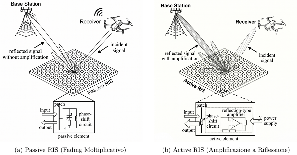
Figura 4: Confronto architetturale tra Reconfigurable Intelligent Surfaces. (a) La propagazione passiva limitata dall’attenuazione moltiplicativa. (b) L’architettura attiva con micro-amplificatori per la mitigazione del path loss.
