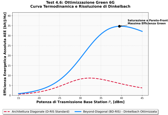
Figura 22: Test 4. Analisi d'Efficienza Energetica Assoluta (AEE). La stima termodinamica dimostra tangibilmente il picco operativo ricercato da Dinkelbach: l'algoritmo scala all'aumentare di P_s fino a saturare il break-even di sistema, esaltando notevolmente il margine di efficienza rate/power per l'avanzato pannello BD-RIS rispetto al subottimale passivo D-RIS standardizzato.
