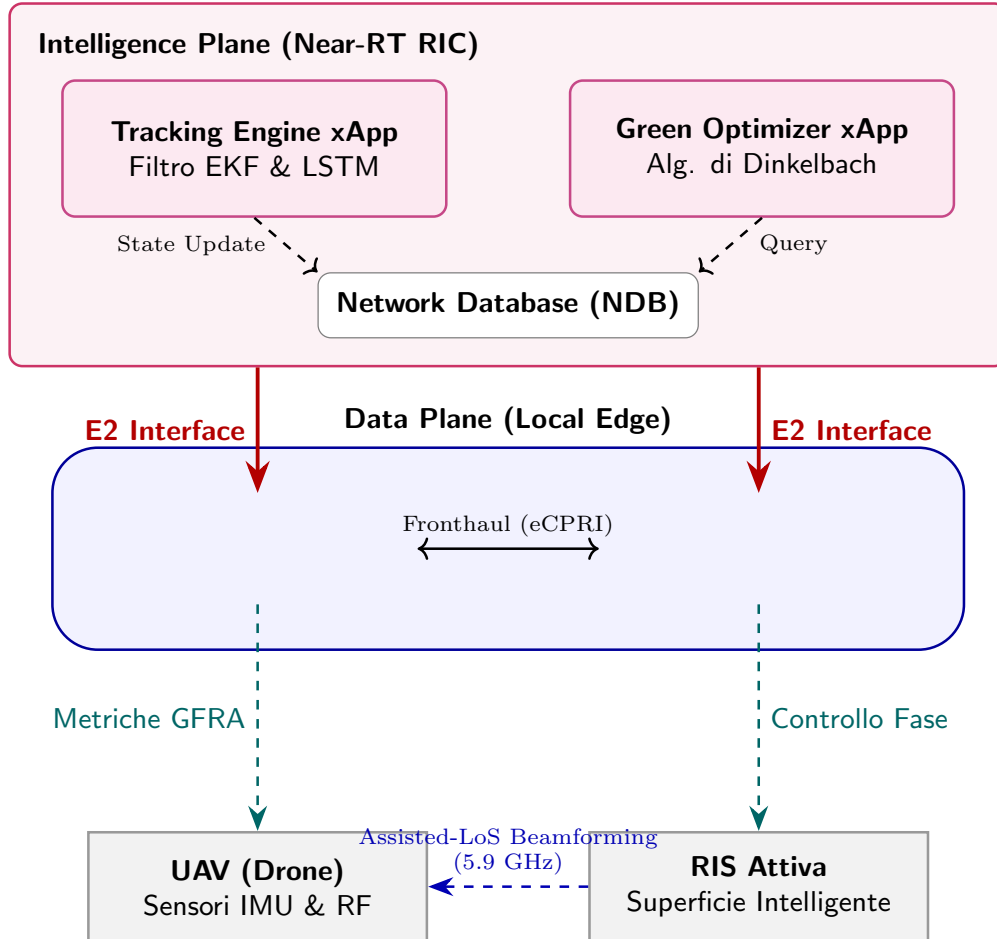
Figura 5: Architettura gerarchica 6G O-RAN. Il piano logico-decisionale (Intelligence Plane) è isolato nell'infrastruttura di rete centrale tramite il nodo Near-RT RIC, comunicando in tempo reale mediante il protocollo standard E2 con le interfacce trasmissive O-DU e O-RU (Data Plane periferico). Questo disaccoppiamento virtualizza gli algoritmi EKF, LSTM e l'ottimizzazione di Dinkelbach sotto forma di xApp native, sollevando interamente il drone (UAV) dai colli di bottiglia computazionali che comprometterebbero l'efficienza energetica della flotta.
