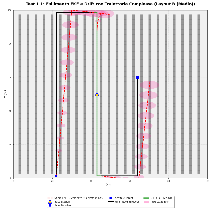
Figura 12: Test 1 (Layout B). Divergenza della traiettoria stimata dall'EKF e logica Coasting.
