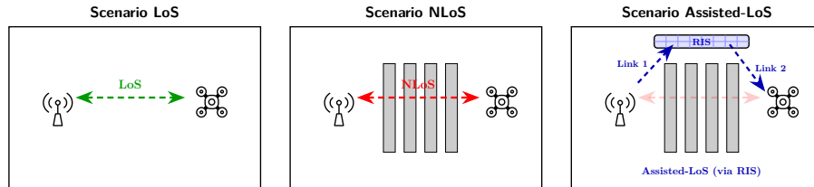
Figura 2: Confronto schematico tra condizione di visibilità diretta (LoS) e ostruzione totale (NLoS) in ambiente industriale magazzino.
