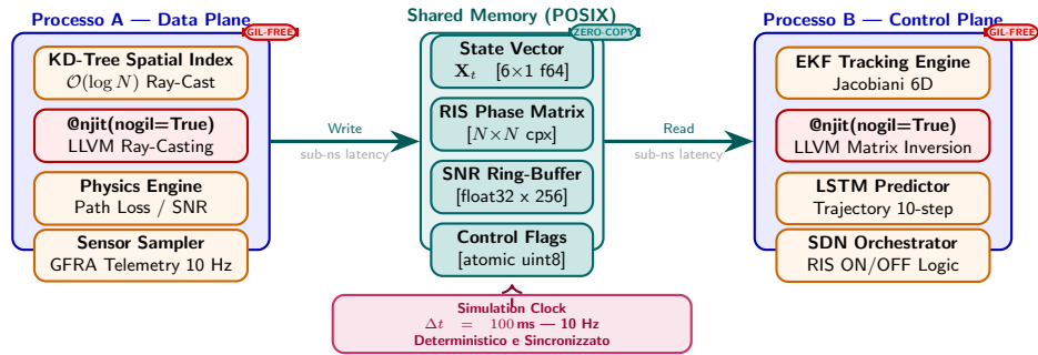
Figura 8: Architettura Software del Digital Twin: Bypass del GIL tramite Multiprocessing e comunicazione Zero-Copy. Il Processo A (Data Plane) esegue il Ray-Casting vettorializzato con KD-Tree e compilazione JIT Numba. Il Processo B (Control Plane) aggiorna le matrici EKF e orchestra le predizioni LSTM. I due processi condividono tensori di stato tramite un segmento POSIX Shared Memory ad accesso diretto (Zero-Copy), azzerando la latenza IPC convenzionale.
