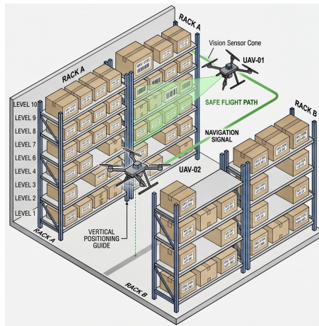
Figura 6: Operazioni di volo e tracciamento multi-UAV.
