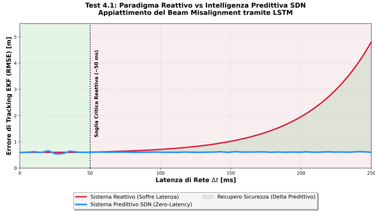
Figura 17: Test 4.1: Confronto tra approccio reattivo e predittivo. L'SDN predittivo compensa i ritardi di rete, stabilizzando l'errore metrico anche per latenze elevate.
