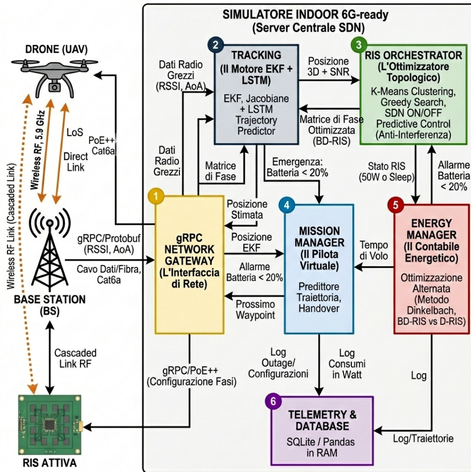
Figura 9: Dettaglio dell'Architettura Logica del Server Centrale SDN e dei suoi macro-moduli interni.
