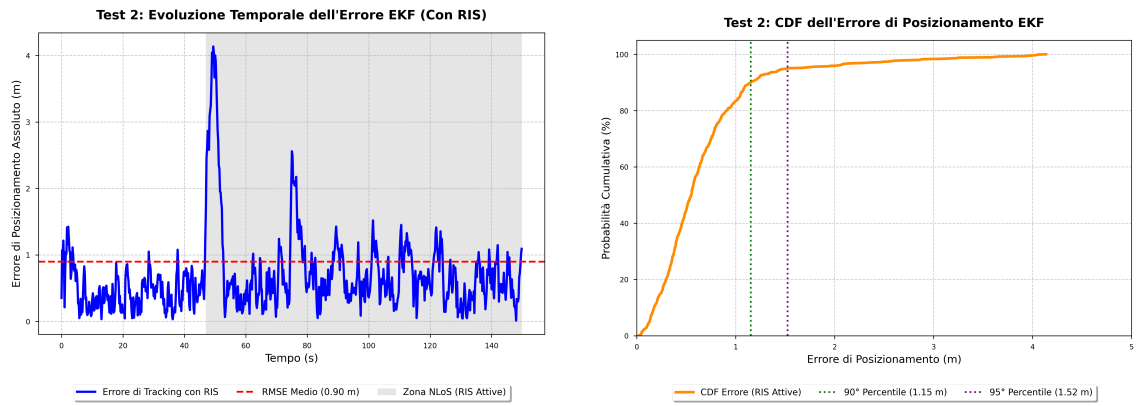
(a) Andamento temporale dell'errore RMSE: ripristino della precisione sub-metrica.
