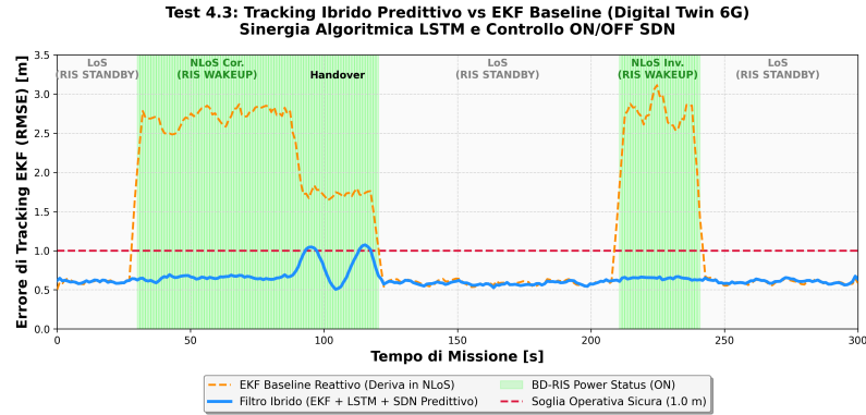
Figura 19: Test 4. L'Analisi Dinamica e Cronologica dell'Errore RMSE. In profilazione comparativa mission-run , lo stimatore standard (Baseline EKF) denuncia severe perdite inerziali in corrispondenza dei varchi NLoS. La stima pilotata in predizione neurale ed assistita dall'SDN (Filtro Ibrido EKF+LSTM) minimizza drasticamente ed ingloba d'autorevolezza gli spike , sigillando la tenuta cinematica in perfetta safe-zone.
