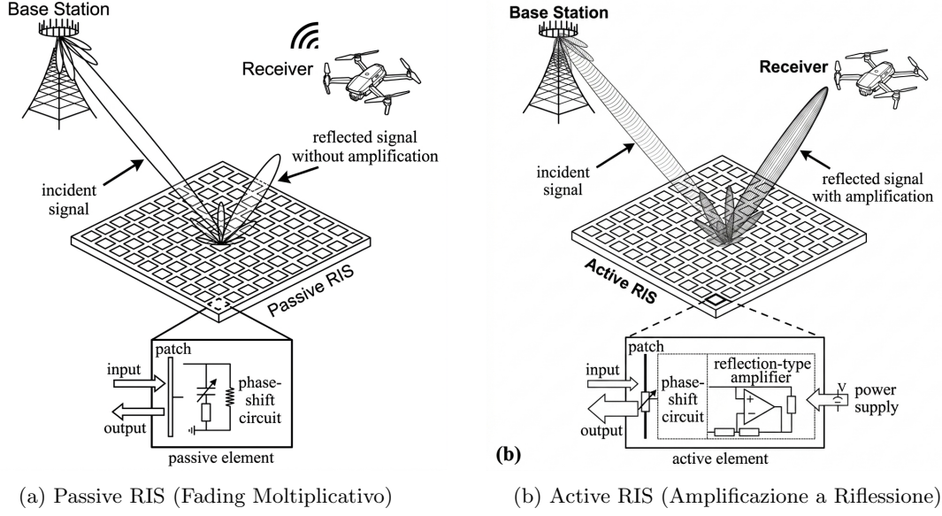
Figura 3: Confronto architetturico tra Reconfigurable Intelligent Surfaces. (a) La propagazione passiva limitata dall'attenuazione moltiplicativa. (b) L'architettura attiva con micro-amplificatori per la mitigazione del path loss.
