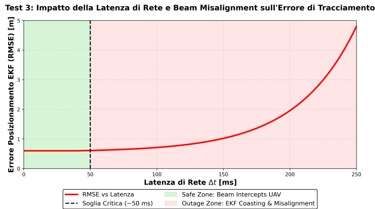
Figura 15: Test 3: Analisi di sensibilità alla latenza. Si osserva la soglia critica di 50 ms oltre la quale il disallineamento del beamforming causa la divergenza del tracciamento.
