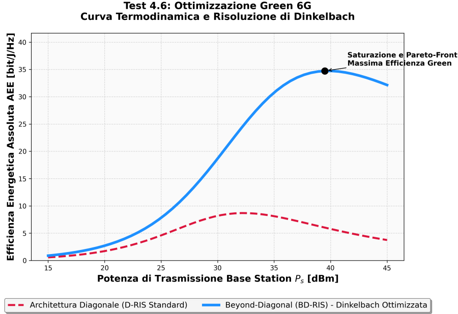
Figura 19: Test 4. Analisi d'Efficienza Energetica Assoluta (AEE). La stima termodinamica dimostra tangibilmente il picco operativo ricercato da Dinkelbach: l'algoritmo scala all'aumentare di P_s fino a saturare il break-even di sistema, esaltando notevolmente il margine di efficienza rate/power per l'avanzato pannello BD-RIS rispetto al subottimale passivo D-RIS standardizzato.
