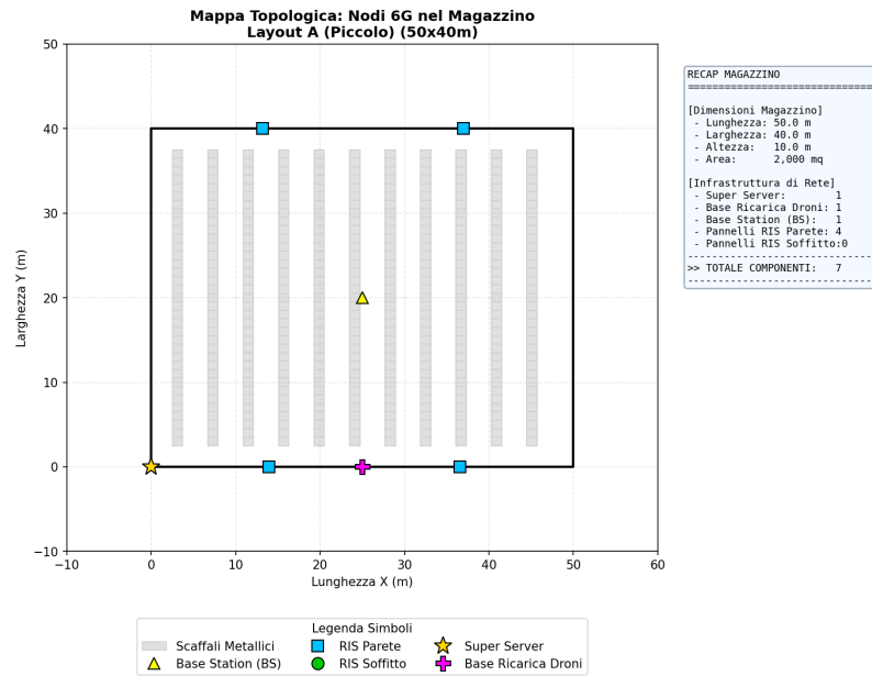
Figura 4: Layout A (50x40m, 4 RIS)
