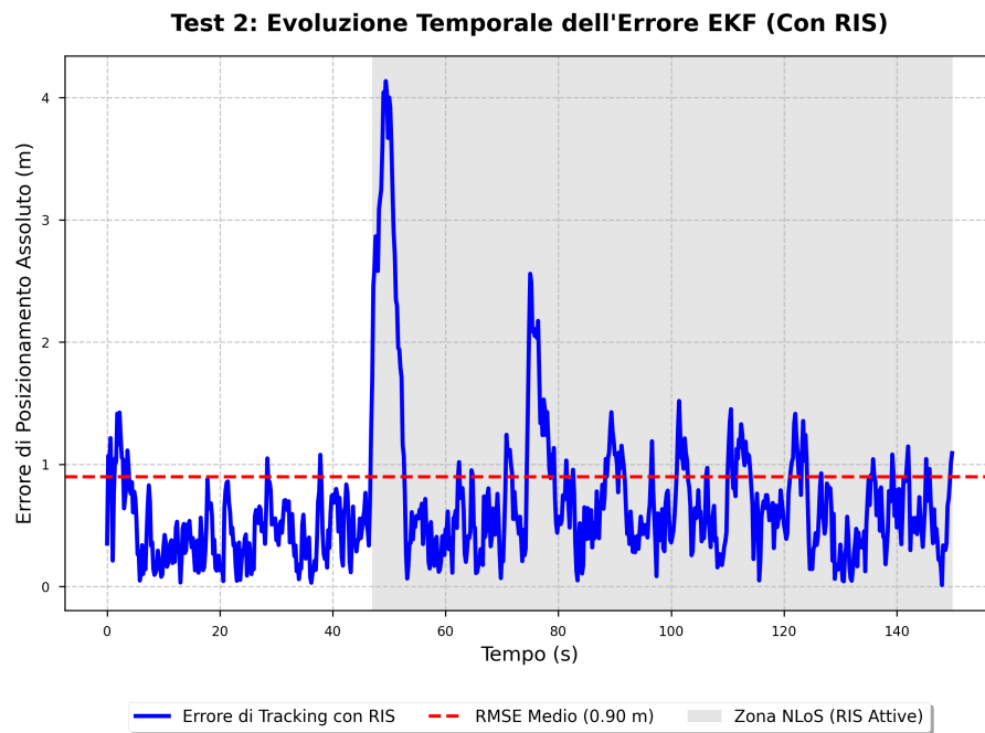
Figura 11: Test 2. Andamento temporale dell'RMSE: l'Assisted-LoS corregge repentinamente la deriva spaziale e mantiene stabile il segnale.
