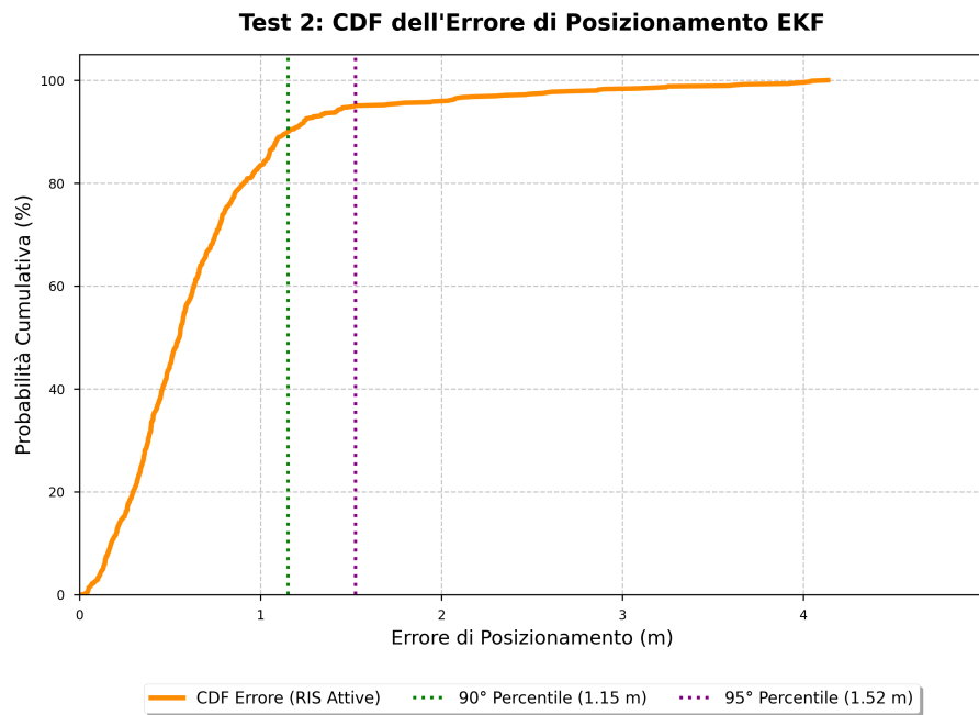
Figura 12: Test 2 (CDF). Valutazione dell'abbattimento della norma dell'errore (RMSE) sotto 1m.
