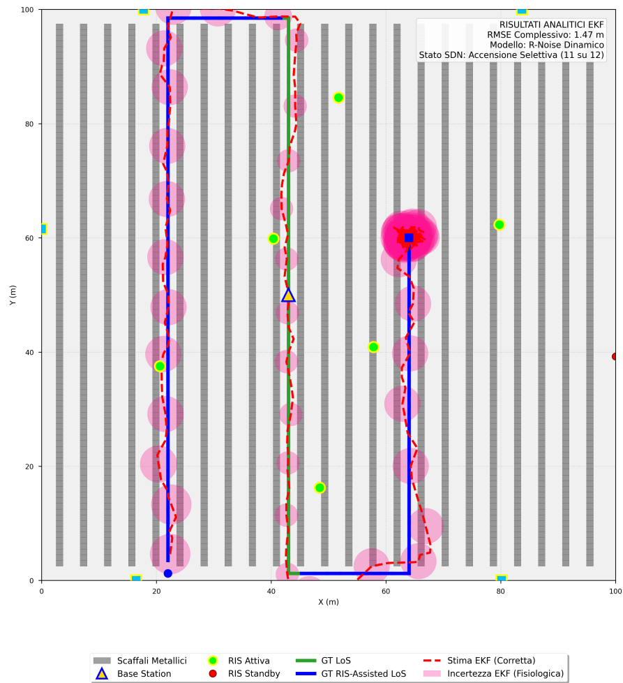
Figura 10: Test 2. Con la RIS attiva per A-LoS interviene il ripristino EKF metrico.
