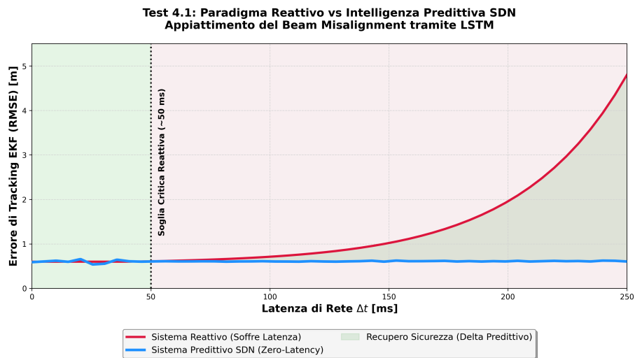
Figura 14: Test 4. Comparativo qualitativo RMSE/Latenza. È documentabile l’appiattimento e l’ammortamento completo del ritardo di trigger operato dall’ingegnerizzazione SDN predittiva contro lo spike disastroso della curva reattiva standardizzata.
