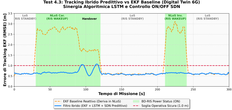
Figura 16: Test 4. L'Analisi Dinamica e Cronologica dell'Errore RMSE. In profilazione comparativa mission-run , lo stimatore standard (Baseline EKF) denuncia severe perdite inerziali in corrispondenza dei varchi NLoS. La stima pilotata in predizione neurale ed assistita dall'SDN (Filtro Ibrido EKF+LSTM) minimizza drasticamente ed ingloba d'autorevolezza gli spike , sigillando la tenuta cinematica in perfetta safe-zone.
