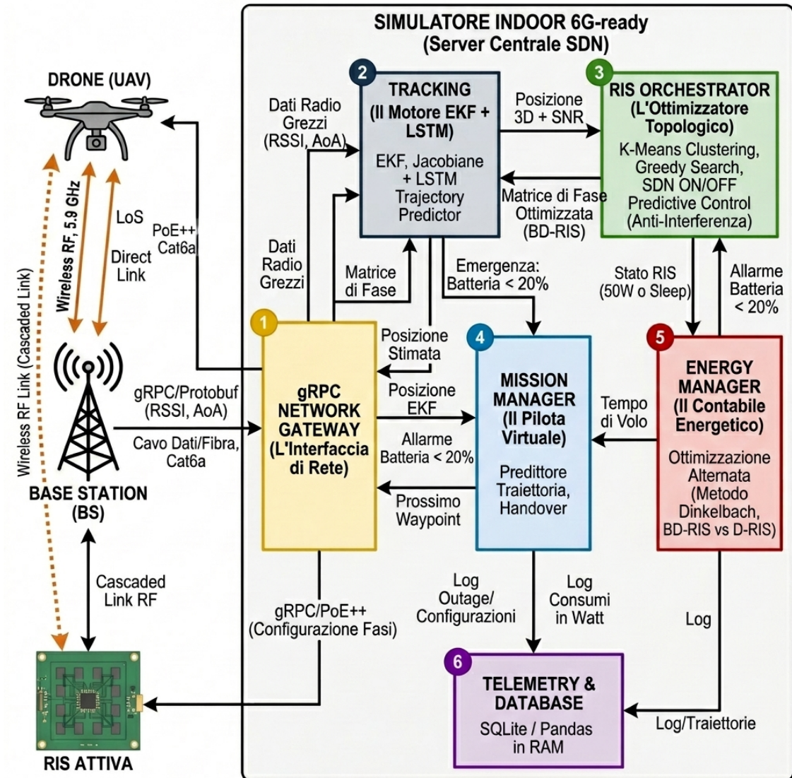
Figura 3: Dettaglio dell'Architettura Logica del Server Centrale SDN e dei suoi macro-moduli interni.
