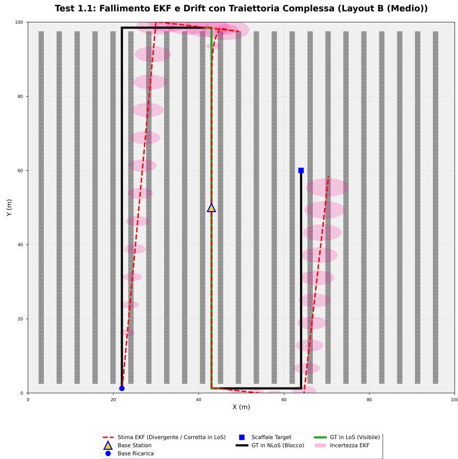
Figura 7: Test 1 (Layout B). Divergenza della traiettoria stimata dall'EKF e logica Coasting.
