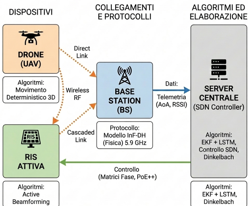
Figura 2: Schema a blocchi semplificato per la separazione dei piani di elaborazione.
