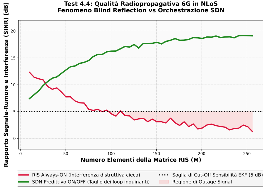
Figura 17: Test 4. Valutazione qualitativa della tolleranza del canale propagativo SINR in densità M . Una configurazione cieca “sempre accesa” tende al collasso del segnale per mutua interferenza, viceversa l’astuta regolazione predittiva ON-OFF dell’SDN protegge e consolida margini stabili di segnale utile bloccati ai limiti Gold-Standard 6G.
