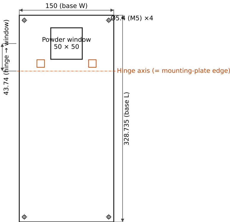
Baseplate — TOP view (Z up out of page)
