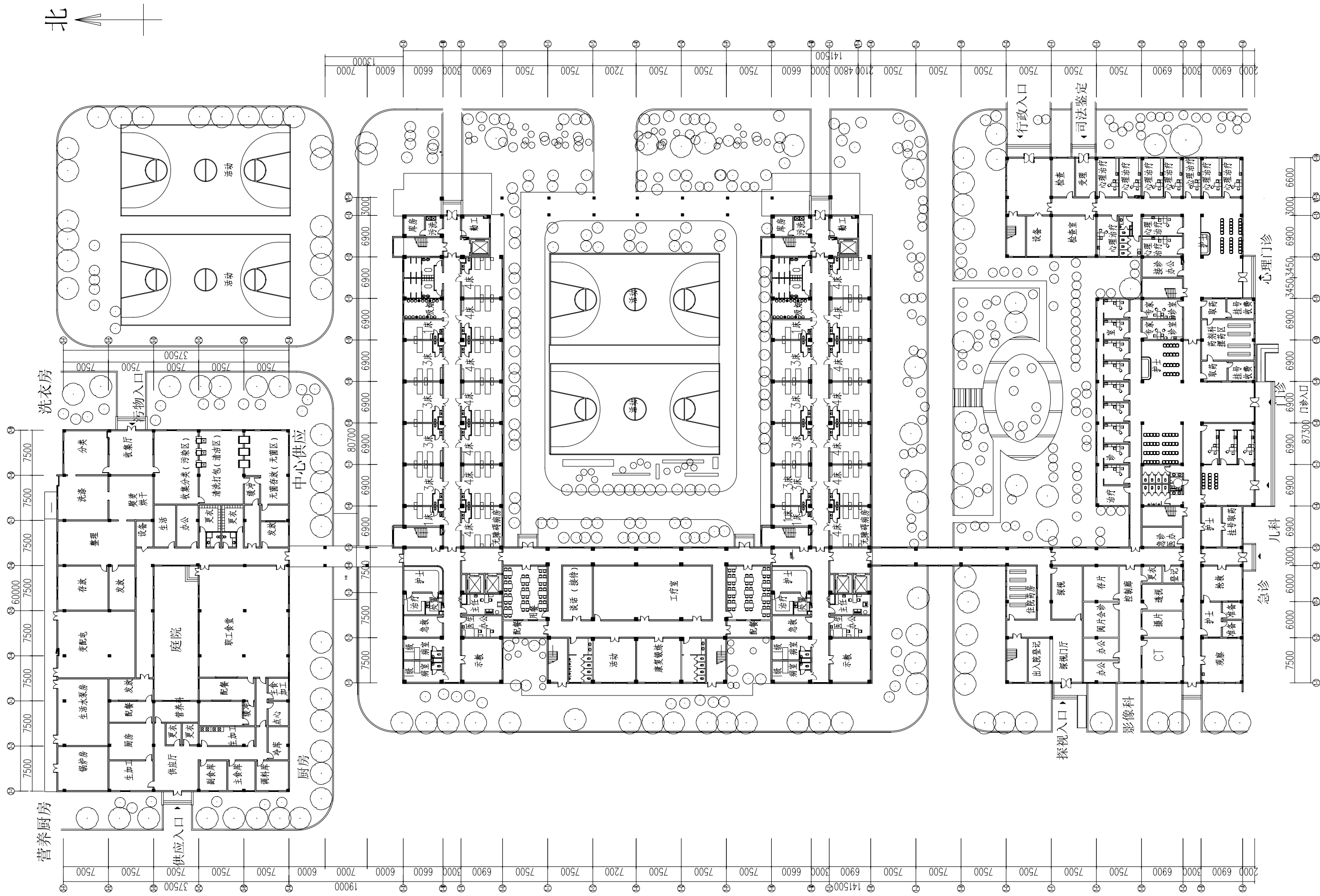
一层平面图 1:600
