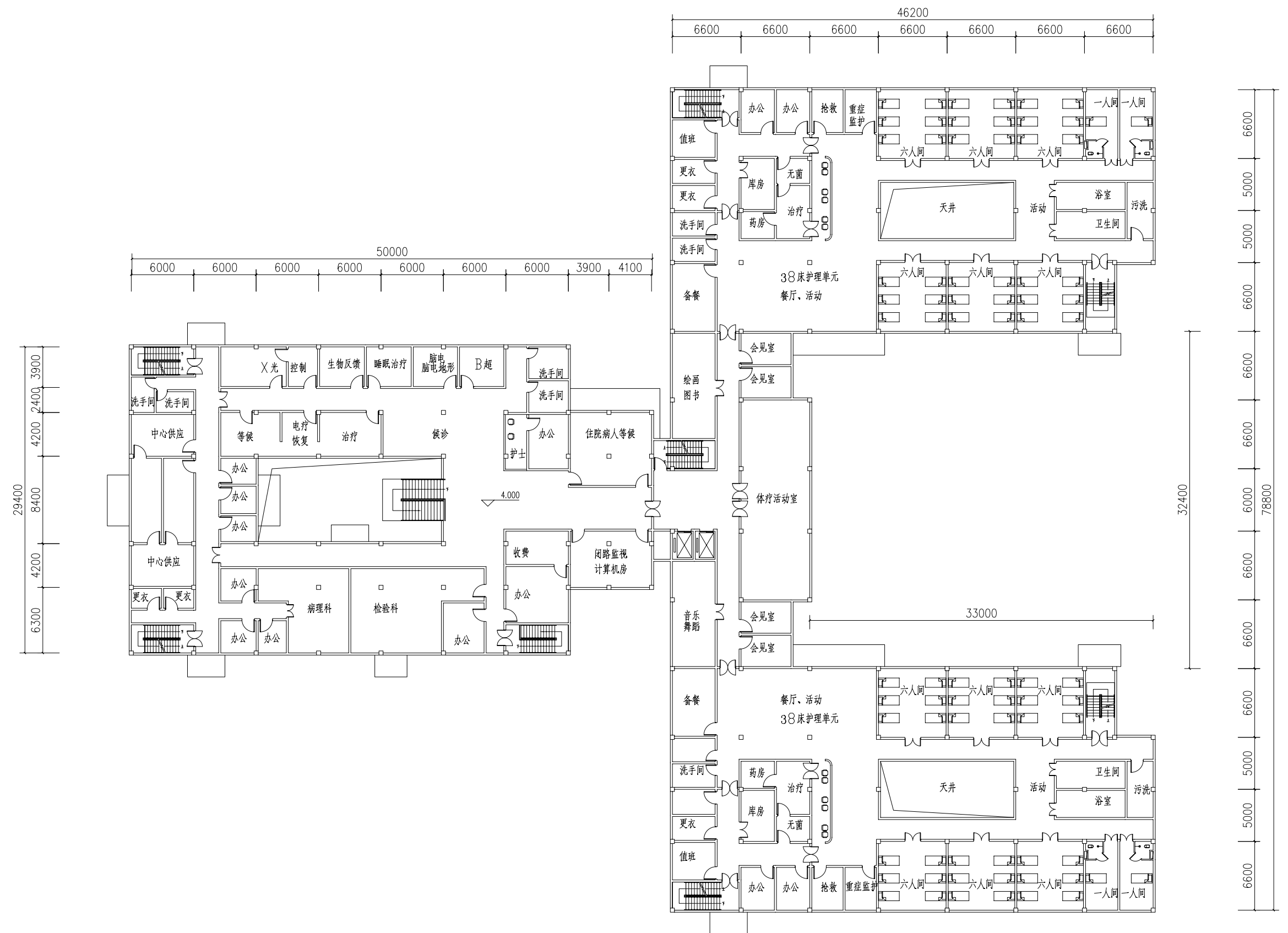
二层平面图 1:400
