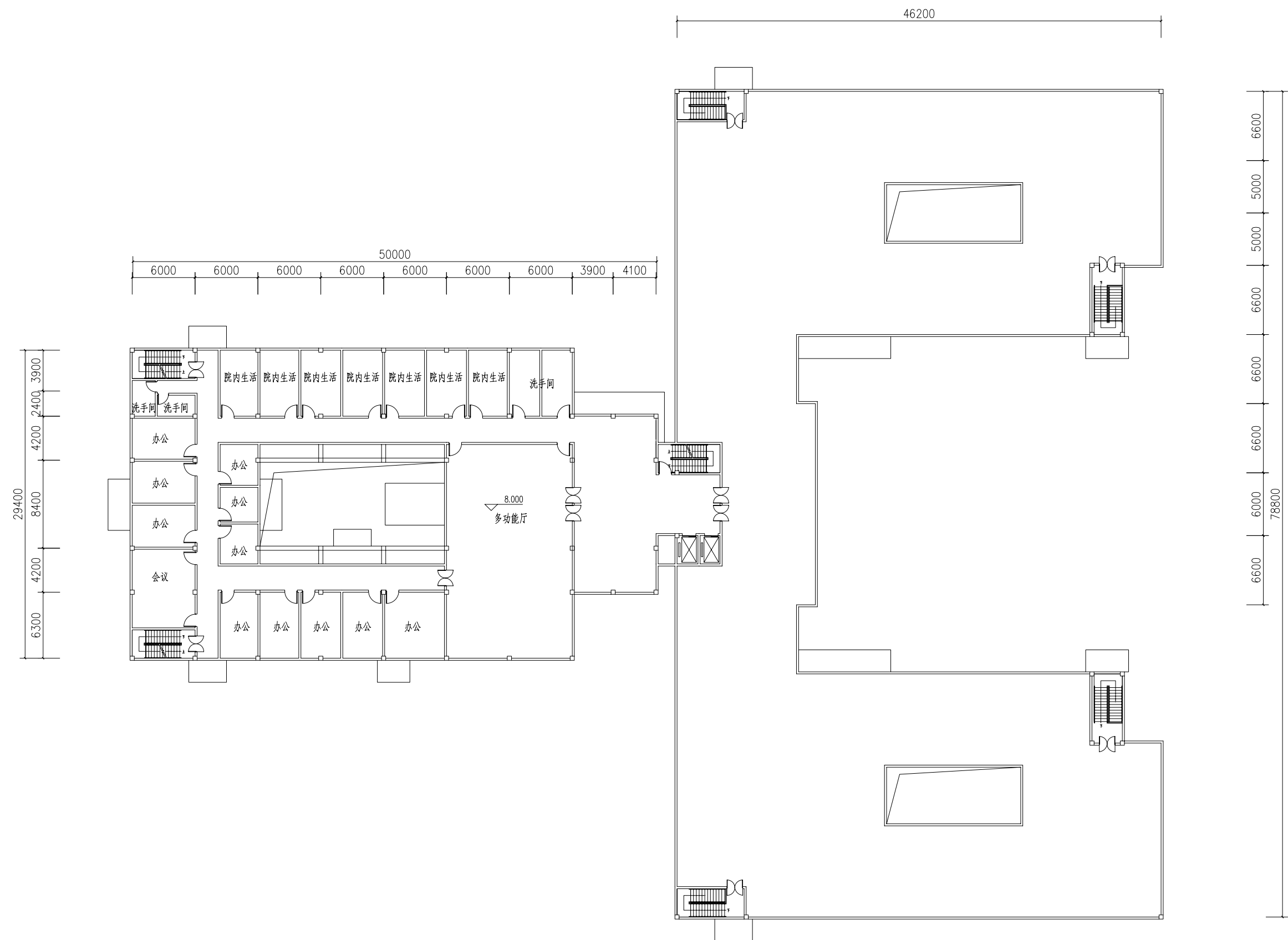
三层平面图 1:400
