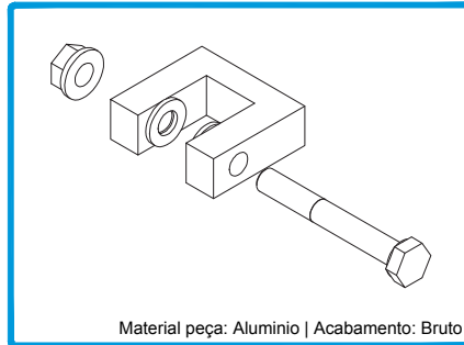
215052 PEÇA FIXAÇÃO EIXO P/ ACIONADOR OR SHAFT FIXING PIECE FOR ACTUATOR PIÈCE DE FIXATION DE L'AXE POUR ACTIONNEUR
