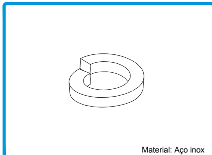
Material: Aço inox 217000 ANILHA MOLA DIN 127 M10 A2 SPRING LOCK WASHER RONDELLE ÉLASTIQUE
