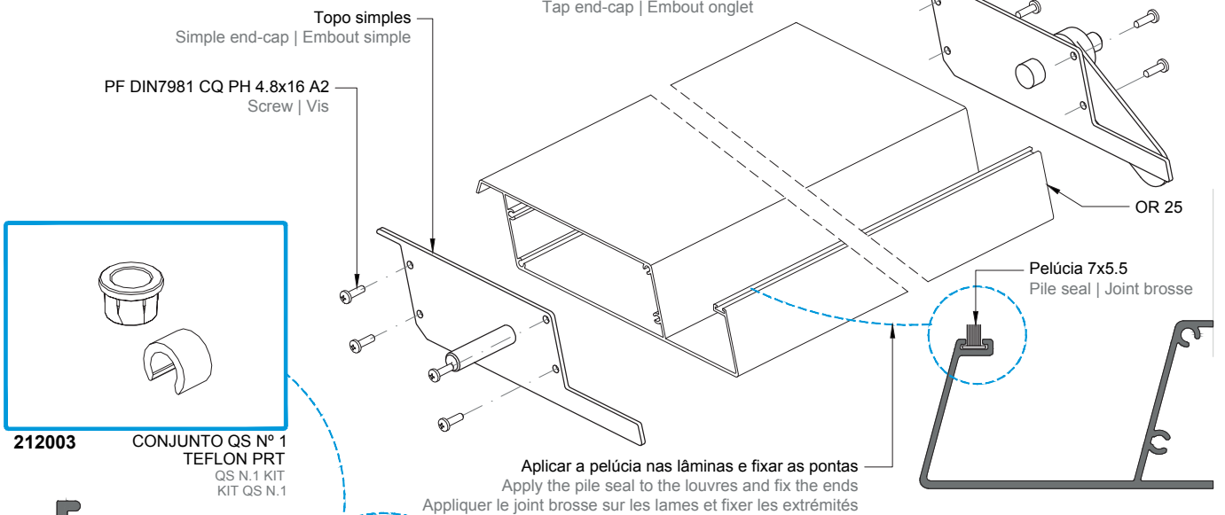
212155 CONJ. TOPOS P/ LAM. MOV. OR25 INOX BRUTO STAINLESS STEEL END CAP KIT KIT D'EMBOUT EN ACIER INOXYDABLE
