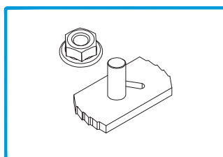
Para fixação do perfil OR 33 ao perfil OR 01 207220 PRESILHA M6x37 CLAMP CLAMEAU
