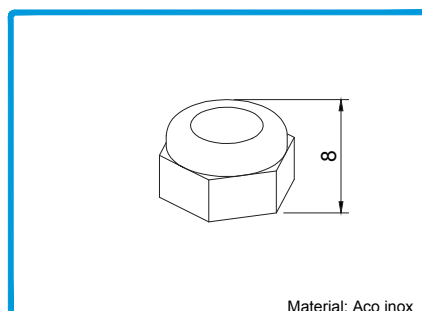
Material: Aço inox 270017 PORCA NYLOC DIN985 M8 A2 NUT HEXAGON WITH NON-METALLIC INSERT ÉCROU À FREIN HEXAGONAL BAGUE NYLON BAS
