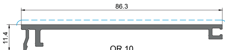
OR 10 Capa (exclusiva para solução orientável e retrátil) Cover (exclusive for orientable and retractable solution) Capot (exclusif pour solution orientable et rétractable)
