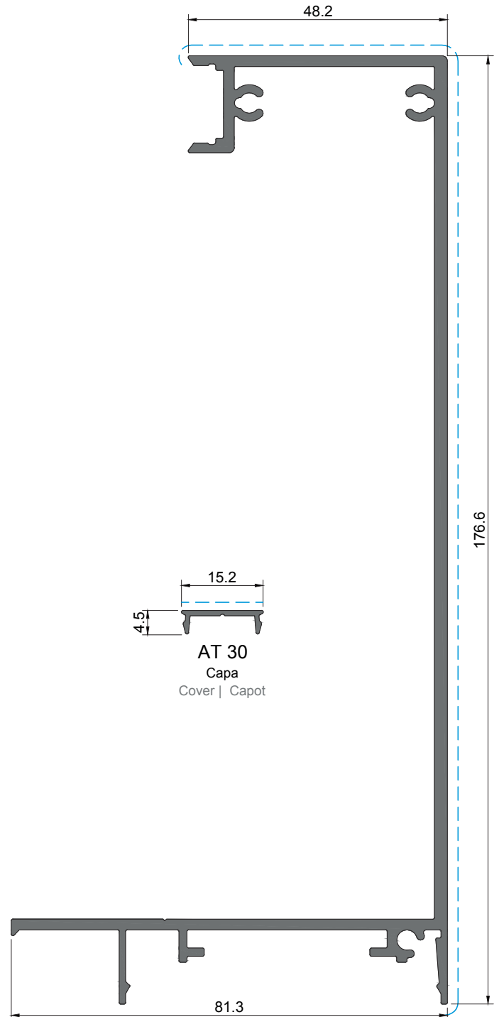
OR 05 Caleira Gutter | Gouttière
