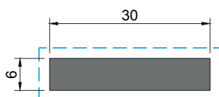
KB 32 Barra (exclusivamente anodizado) Flat bar (exclusively polished) Barre plates (exclusivement anodisé)
