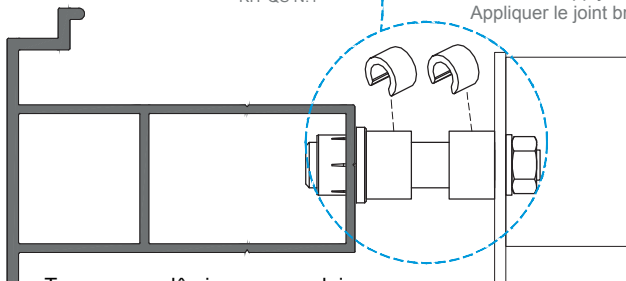
212003 CONJUNTO QS Nº 1 TEFLON PRT QS N.1 KIT KIT QS N.1
