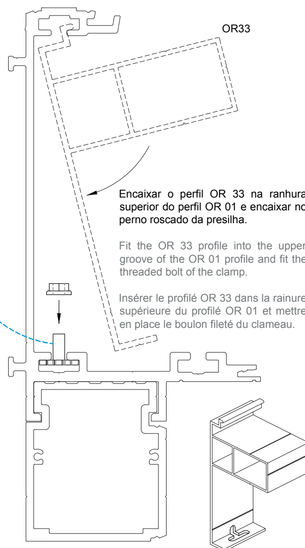
Para fixação do perfil OR 33 ao perfil OR 01 207220 PRESILHA M6x37 CLAMP CLAMEAU
