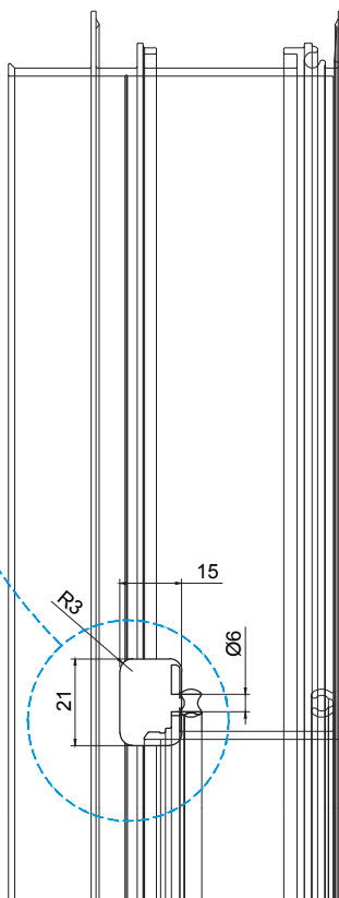
Rasgo para aplicação da Ponte para cabos LED Slot for the application of the LED Cable holder Déchirure pour l'application de Support de câbles
