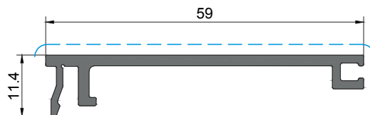
OR 11 Capa (exclusiva para solução orientável e retrátil) Cover (exclusive for orientable and retractable solution) Capot (exclusif pour solution orientable et rétractable)
