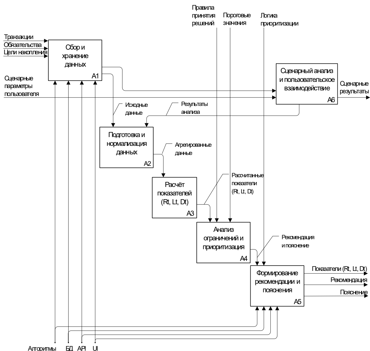
Рисунок 9 – Контекстная диаграмма «ТО BE» декомпозиция A1–A6 (IDEF0)
