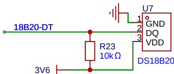
18B20插座
