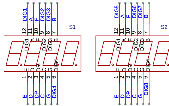
共阴数码管
