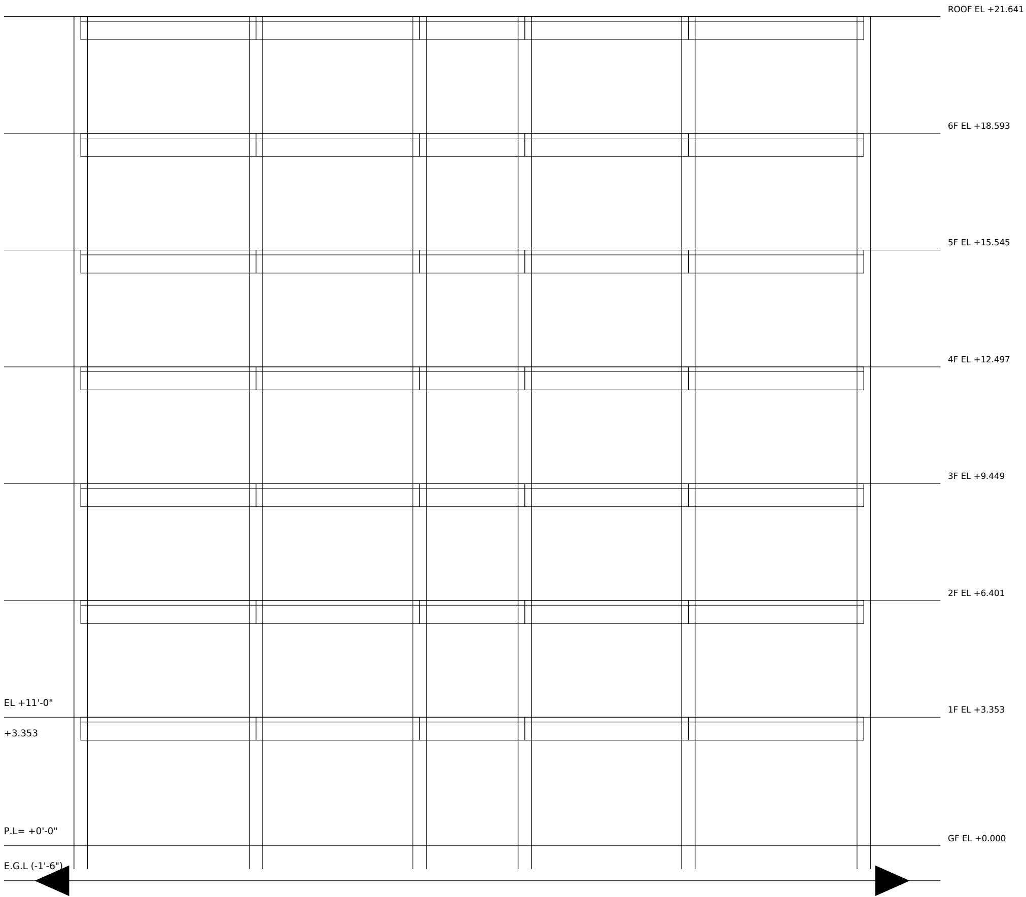
SECTION A-A
