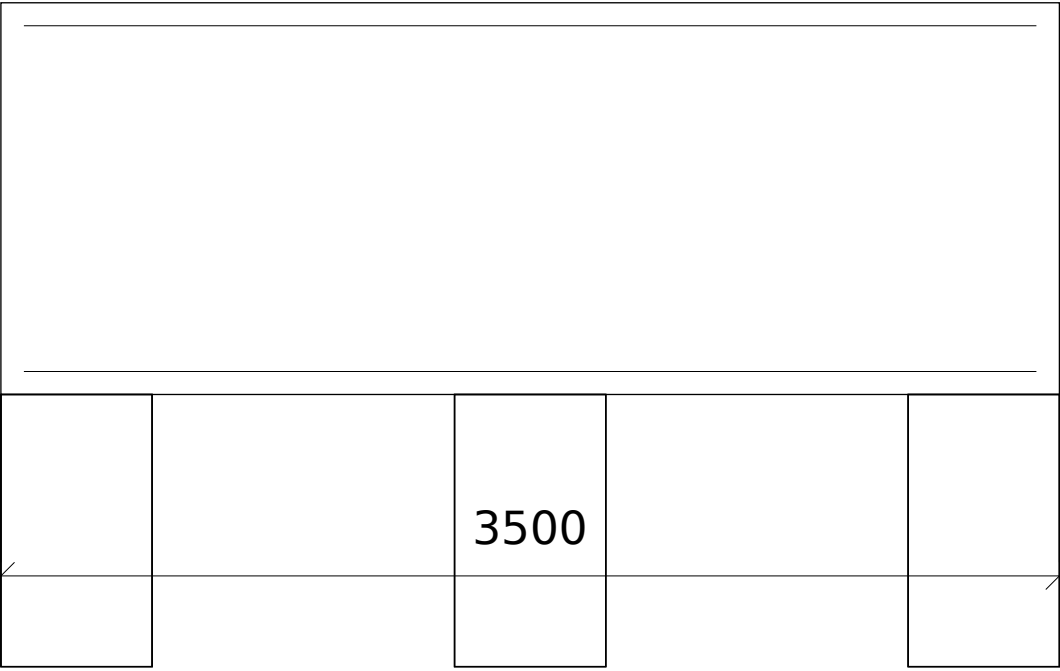
PC5
