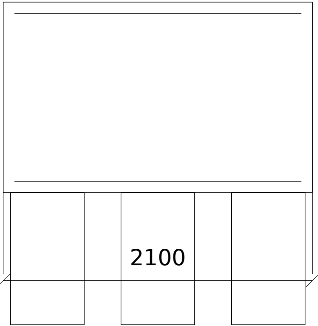
PC2
