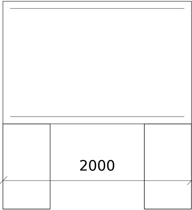
PC3
