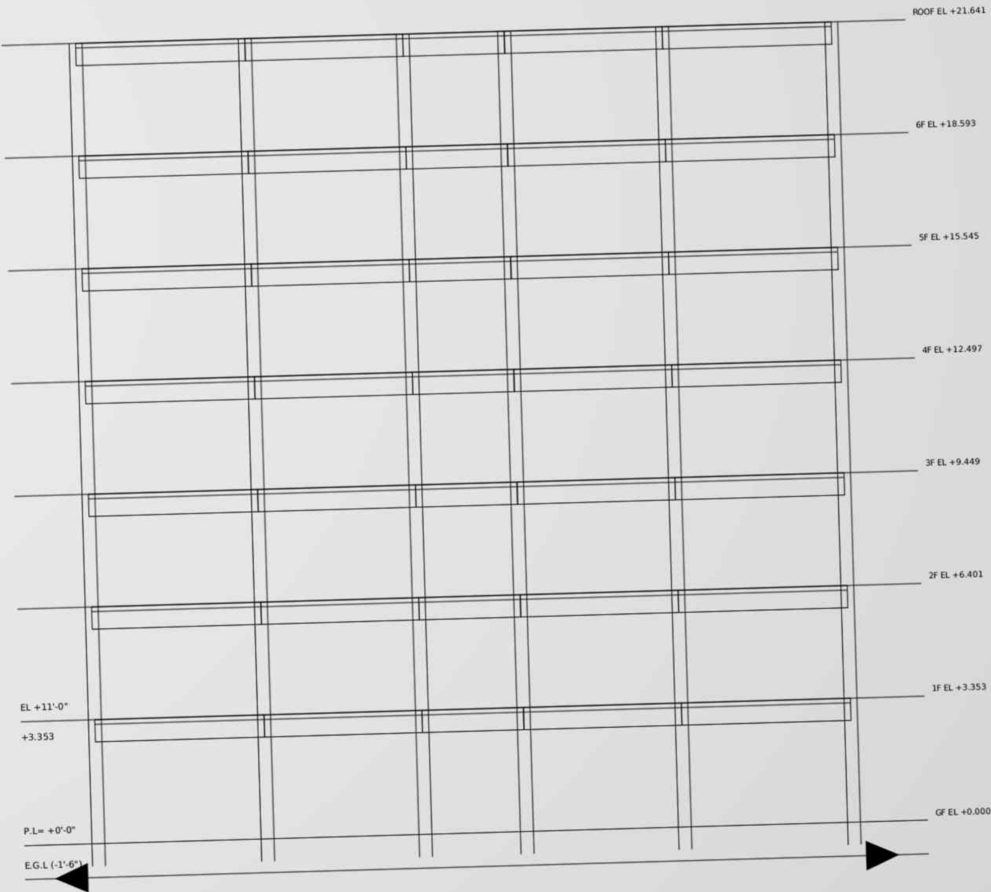
SECTION A-A
