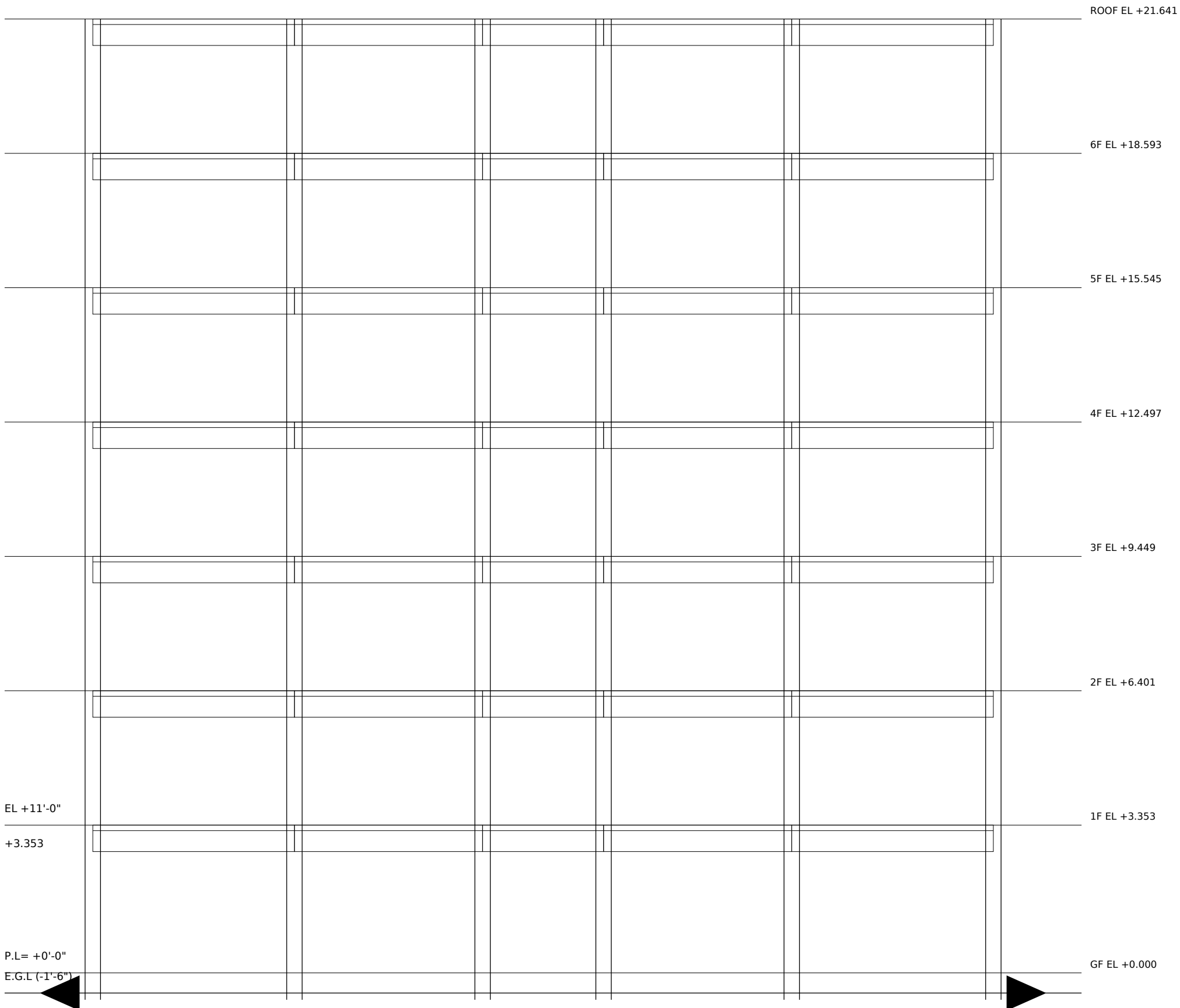
SECTION A-A
