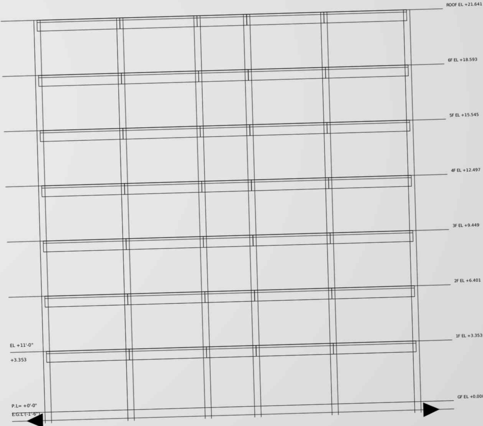
SECTION A-A
