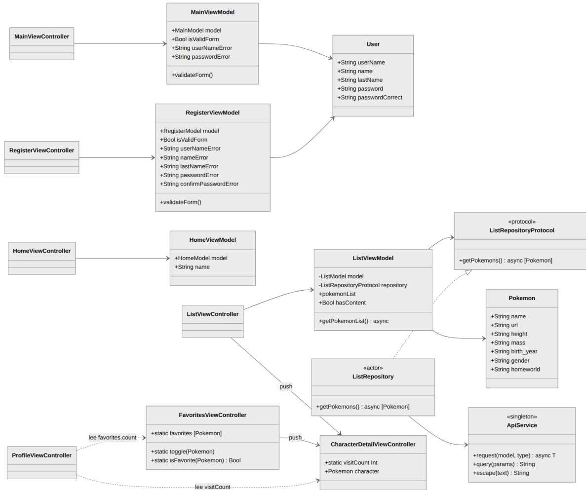
Diagrama de clases (pantallas, lógica y datos separados)
