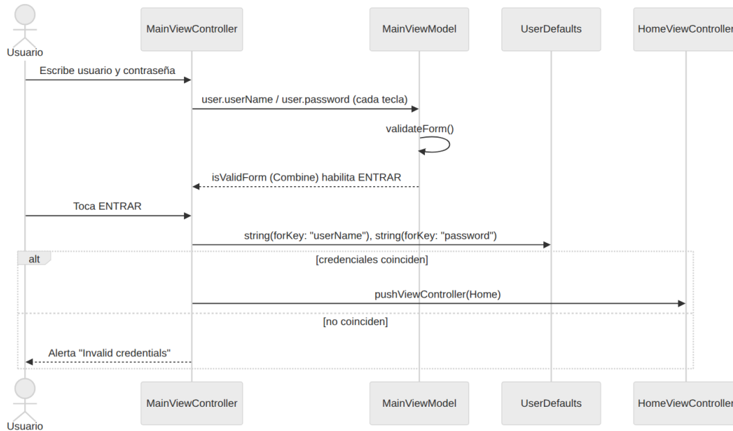
Secuencia del inicio de sesión
