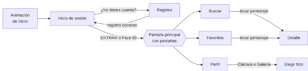
Navegación entre pantallas
