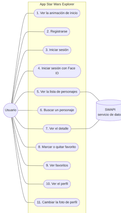
Casos de uso
