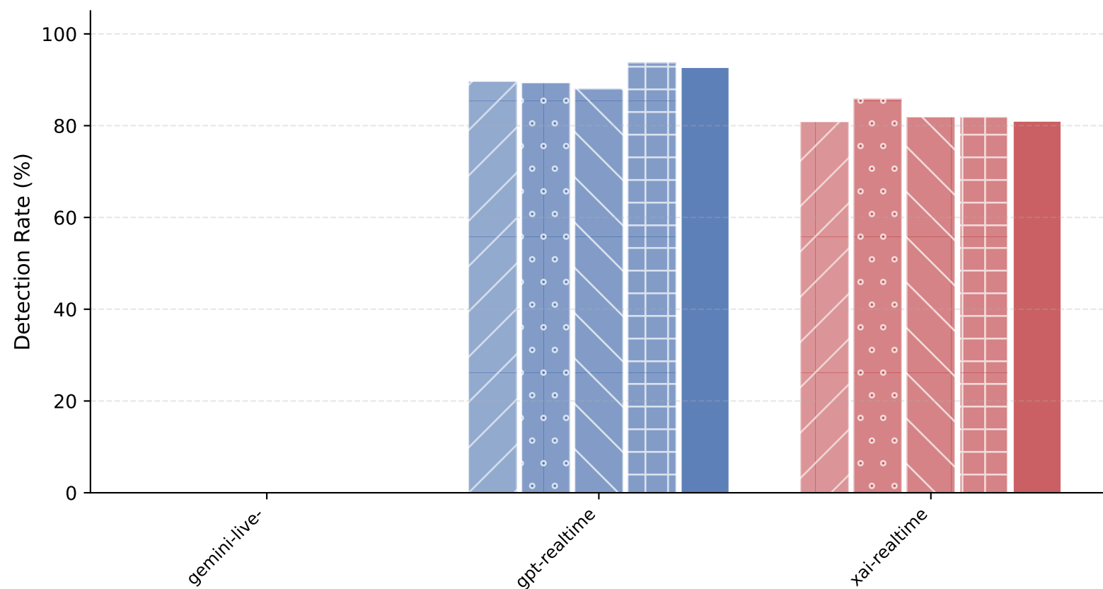
LLM Telecom
