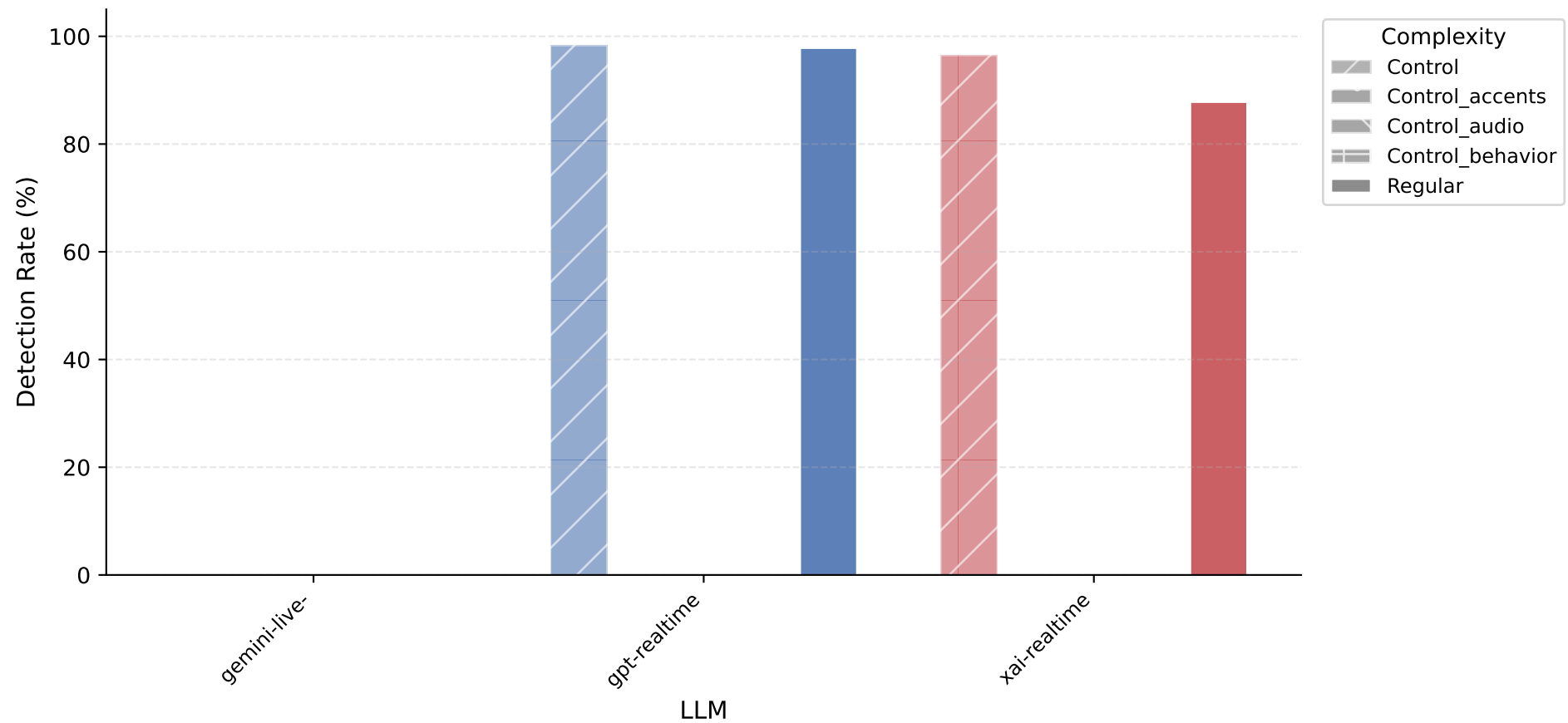
LLM Telecom
