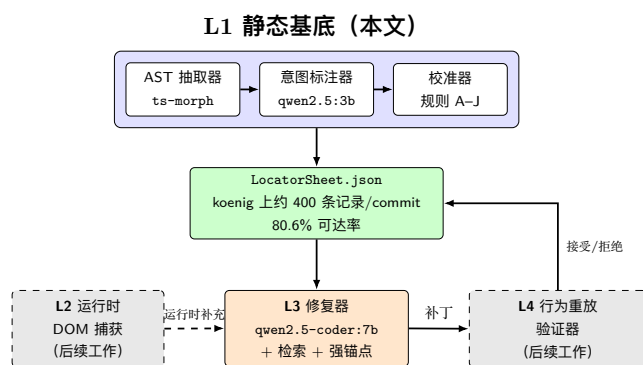
图 1 HealReact 流水线。L1（本文）是静态 AST 锚点基底，意图标注层在本文中仅在 32 元素的小规模构造样例 (fixture) 上评估；L3 是 §3 中评估的 LLM 修复器。L2（运行时 DOM 捕获）与 L4（行为重放验证器 / virtual oracle）以虚线框表示，二者在本文中均为设计占位、留作后续工作：L2 负责静态不可见的运行时元素，L4 的必要性由 §3 中的对抗性误修复探针在经验上得到充分动机化。
