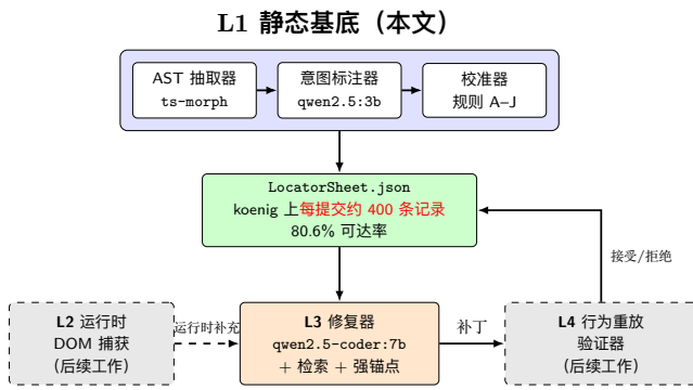
图1 HealReact 流水线。L1（本文）是静态 AST 锚点基底，意图标注层在本文中仅在 32 元素的小规模构造样例集上评估；L3 是 §3 中评估的 LLM 修复器。L2（运行时 DOM 捕获）与 L4（行为重放验证器）以虚线框表示，二者在本文中均为设计占位、留作后续工作：L2 负责静态不可见的运行时元素，L4 的必要性由 §3 中的对抗性误修复探针在经验上得到充分动机化。
