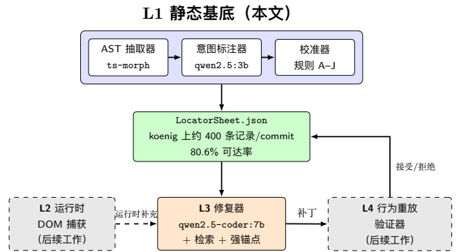
图 1 HealReact 诊断测量平台与未来流水线关系。L1（本文）是静态 AST 锚点基底，意图标注层在本文中仅在 32 元素的小规模构造样例（fixture）上评估；L3 是 §3 中评估的 LLM 修复器。L2（运行时 DOM 捕获）与 L4（行为重放验证器 / virtual oracle）以虚线框表示，二者在本文中均为设计占位、留作后续工作：L2 负责静态不可见的运行时元素，L4 的必要性由 §3 中的对抗性误修复探针在经验上得到充分动机化。
