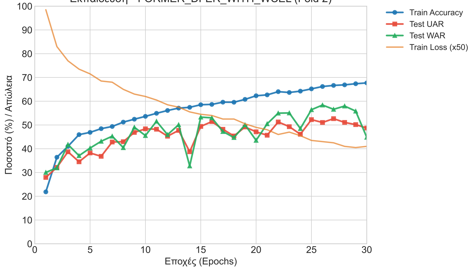
Εκπαίδευση - FORMER_DFER_WITH_WCEL (Fold 2)
