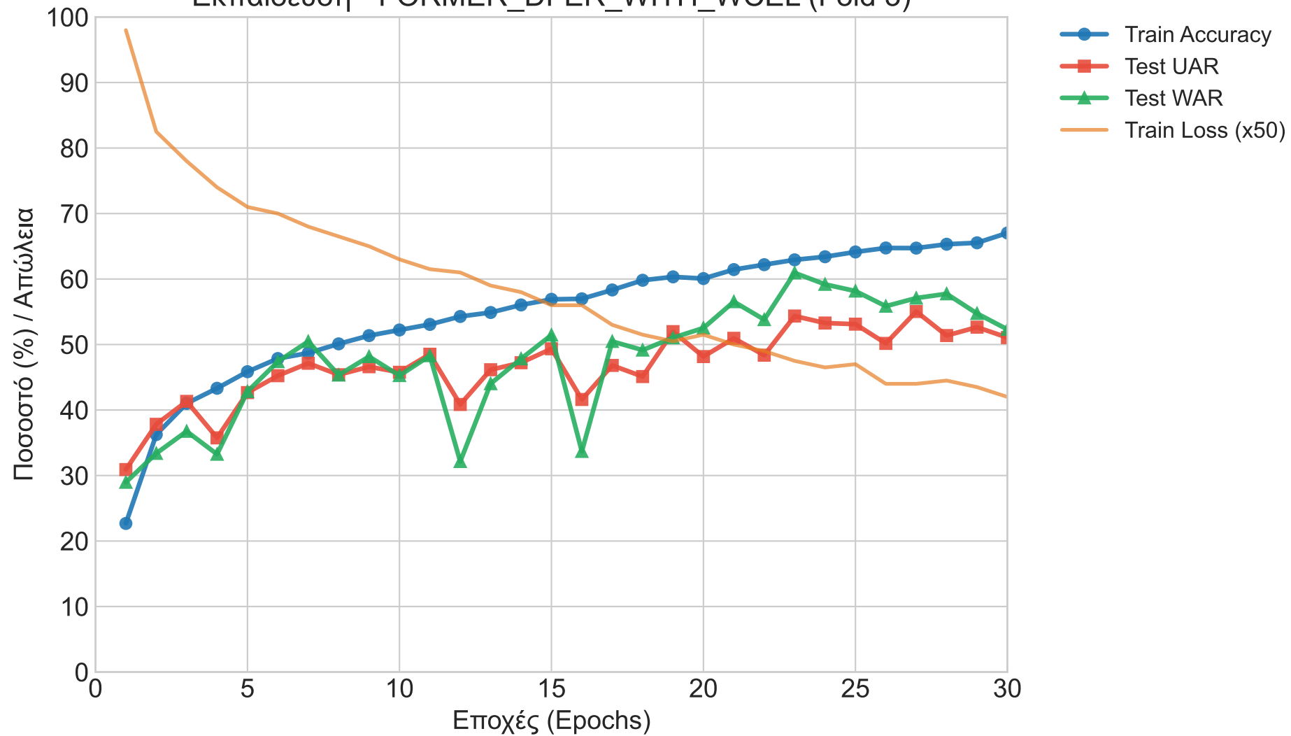
Εκπαίδευση - FORMER_DFER_WITH_WCEL (Fold 3)
