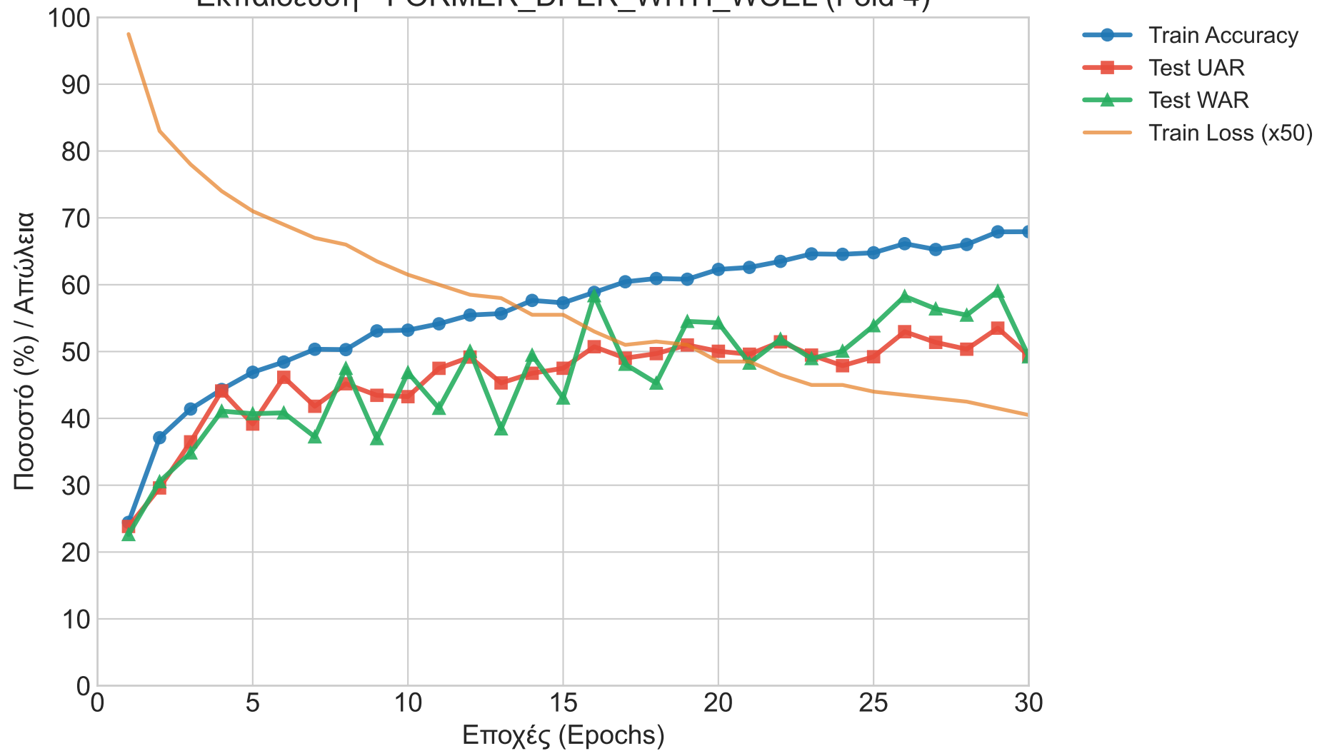
Εκπαίδευση - FORMER_DFER_WITH_WCEL (Fold 4)
