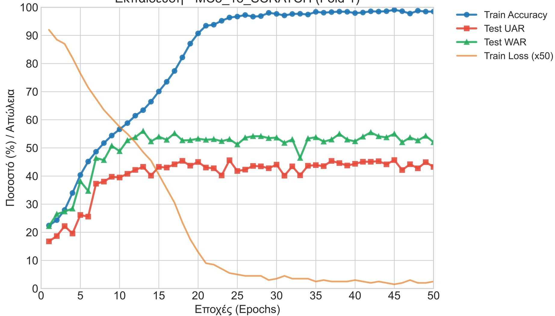
Εκπαίδευση - MC3_18_SCRATCH (Fold 1)
