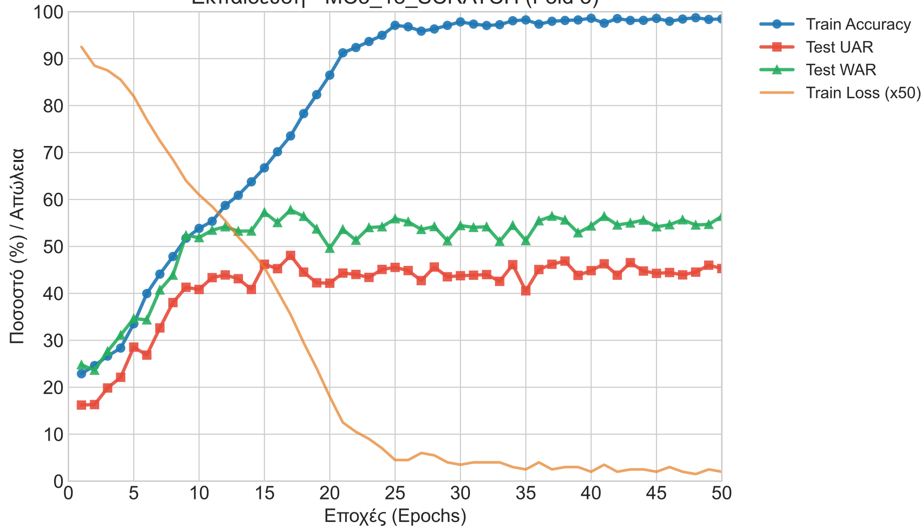
Εκπαίδευση - MC3_18_SCRATCH (Fold 3)
