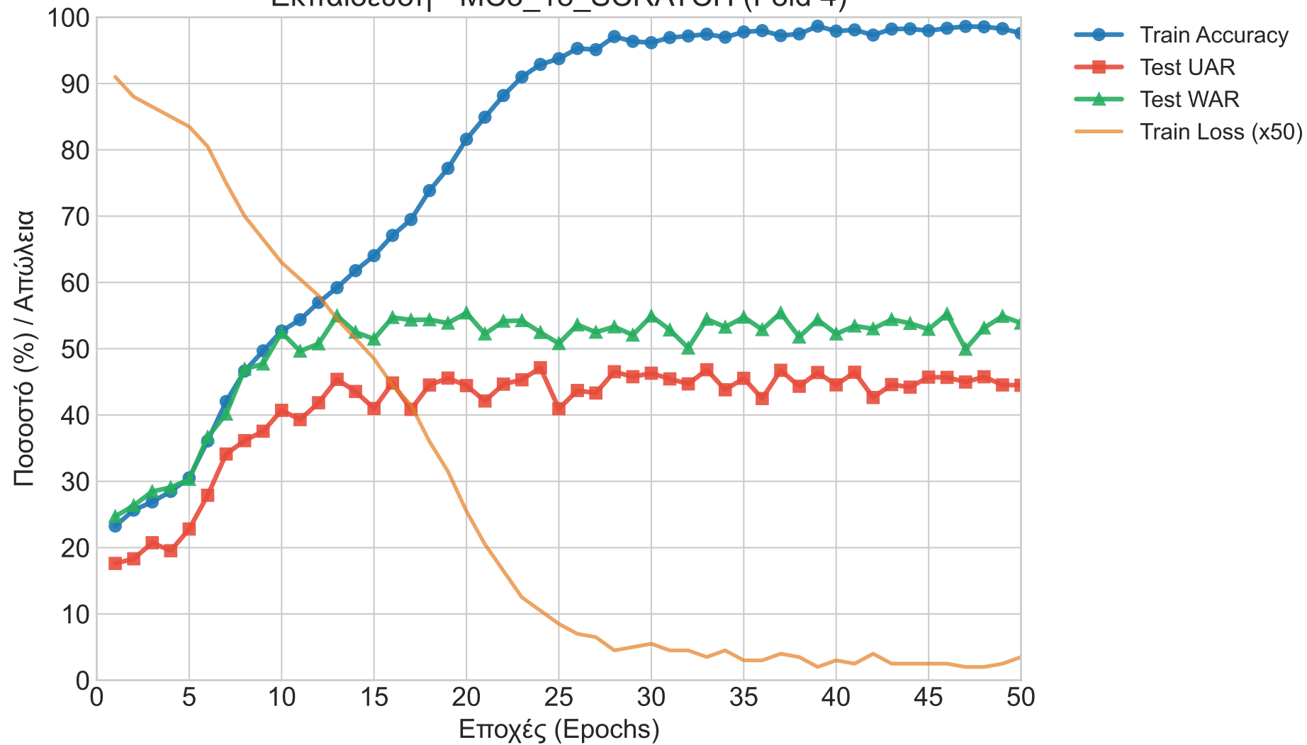
Εκπαίδευση - MC3_18_SCRATCH (Fold 4)
