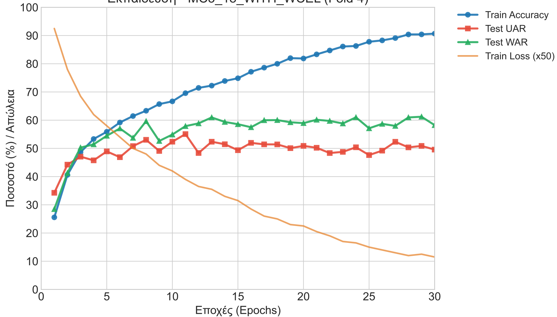
Εκπαίδευση - MC3_18_WITH_WCEL (Fold 4)
