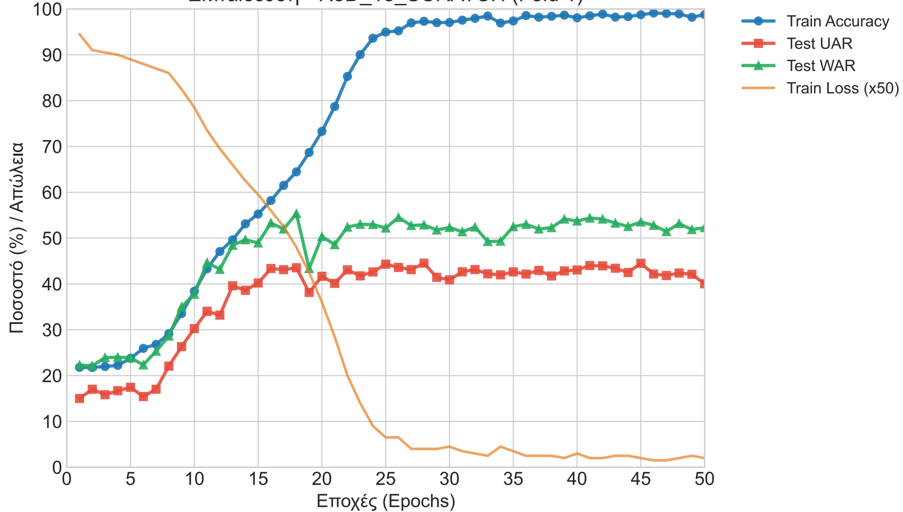
Εκπαίδευση - R3D_18_SCRATCH (Fold 1)
