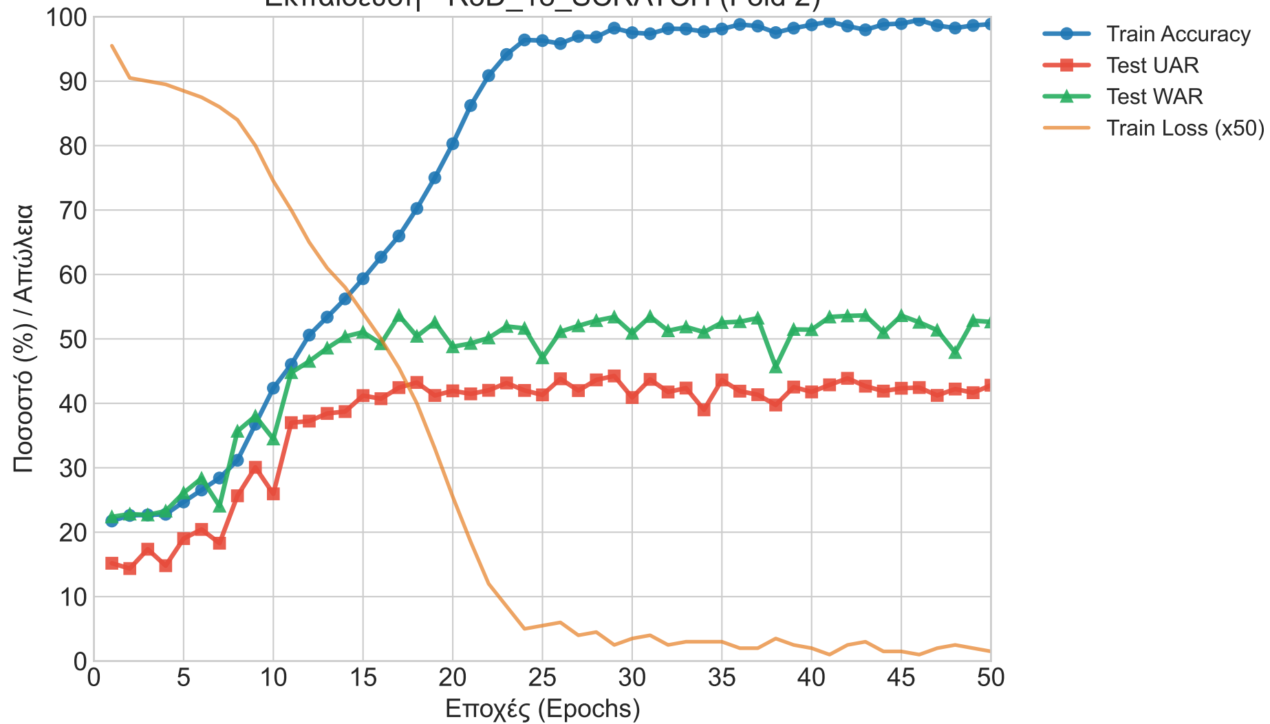
Εκπαίδευση - R3D_18_SCRATCH (Fold 2)
