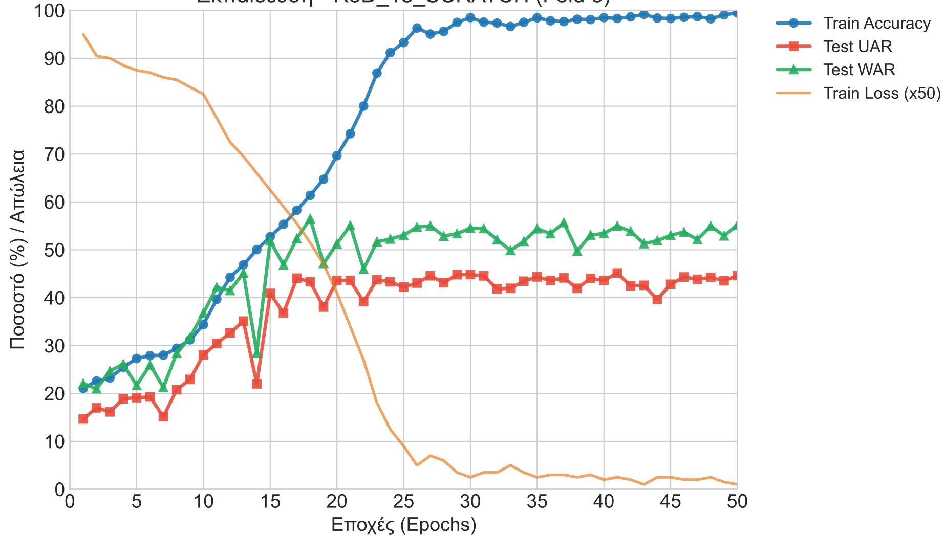
Εκπαίδευση - R3D_18_SCRATCH (Fold 3)
