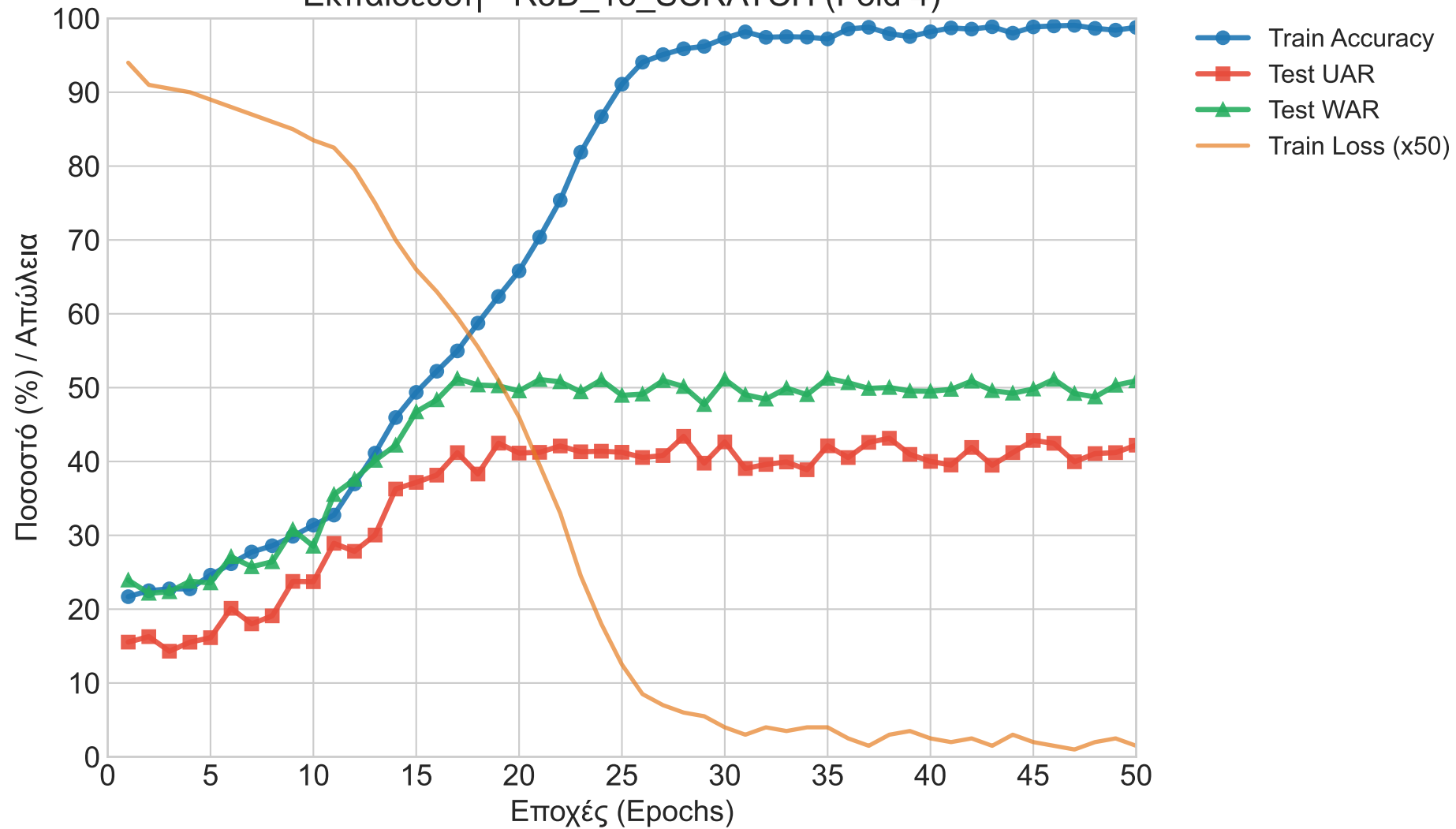
Εκπαίδευση - R3D_18_SCRATCH (Fold 4)
