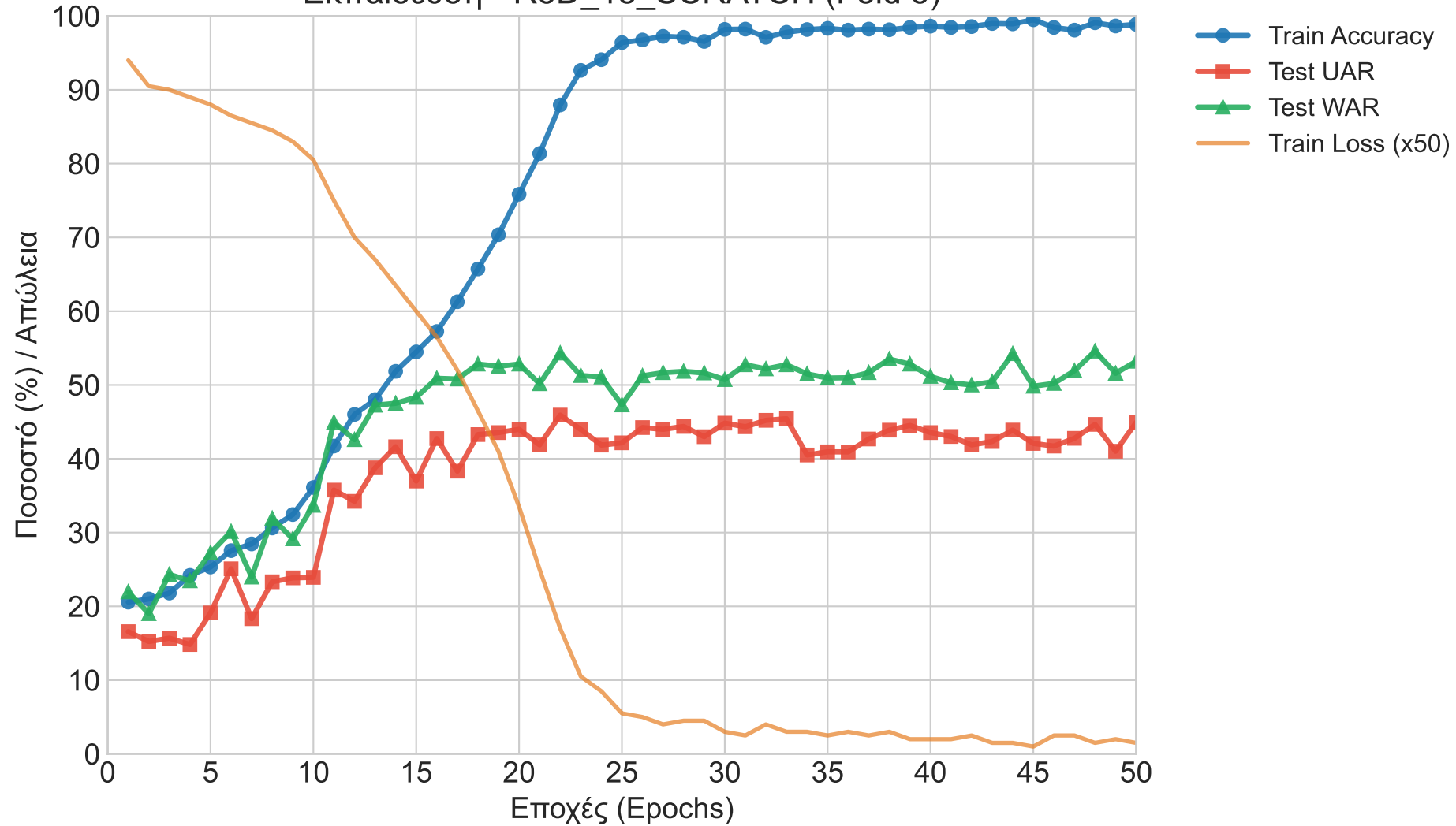
Εκπαίδευση - R3D_18_SCRATCH (Fold 5)
