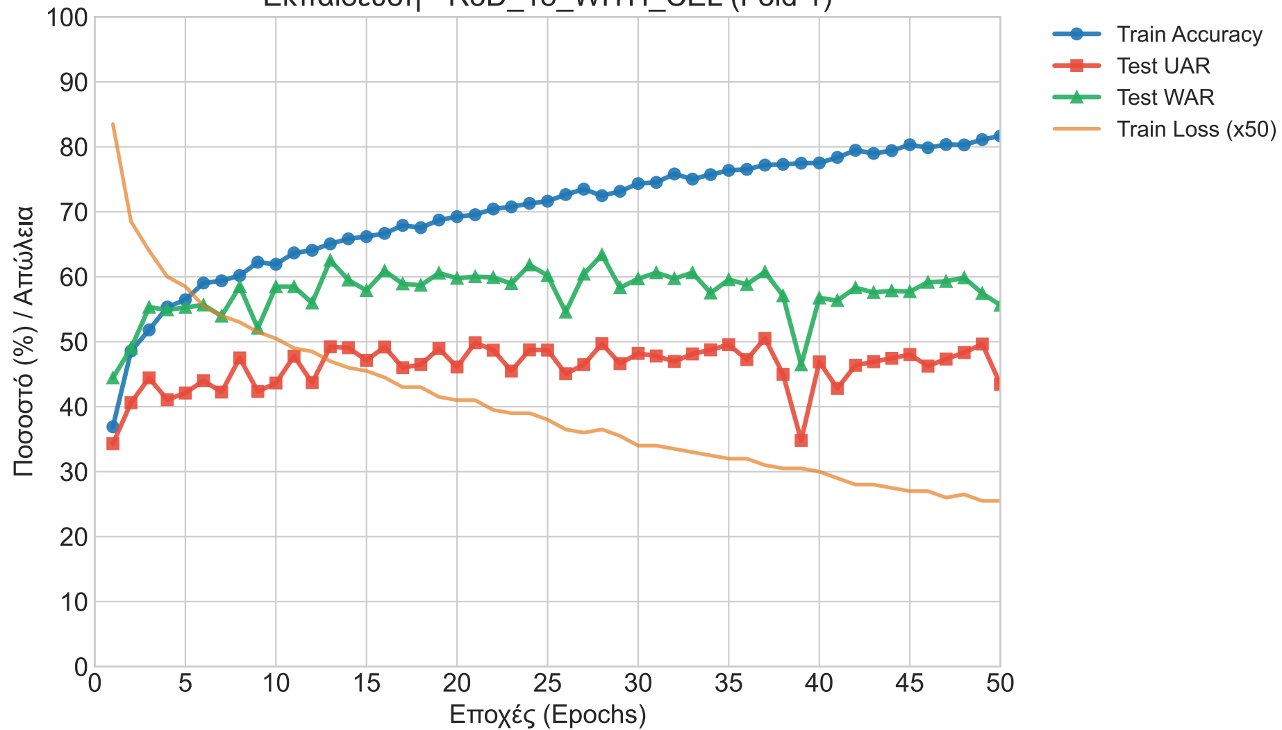
Εκπαίδευση - R3D_18_WITH_CEL (Fold 1)
