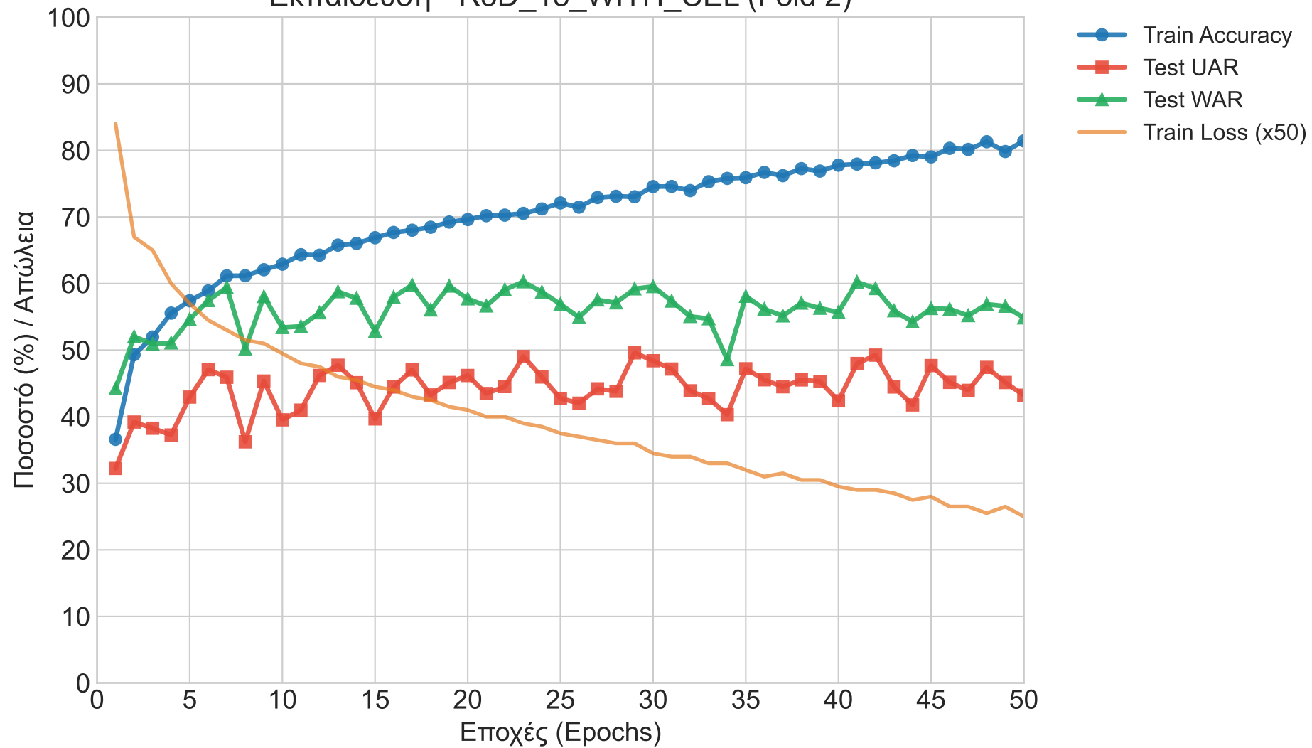
Εκπαίδευση - R3D_18_WITH_CEL (Fold 2)
