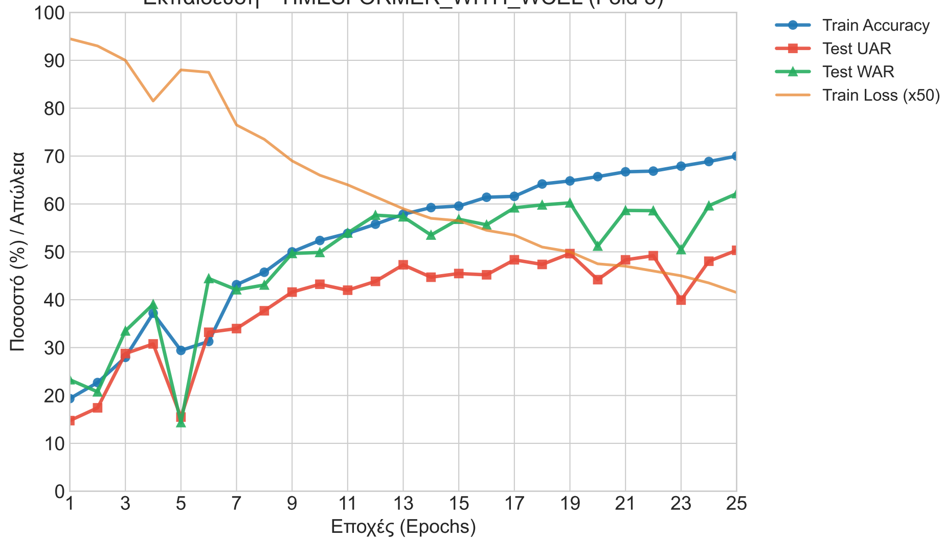
Εκπαίδευση - TIMESFORMER_WITH_WCEL (Fold 5)
