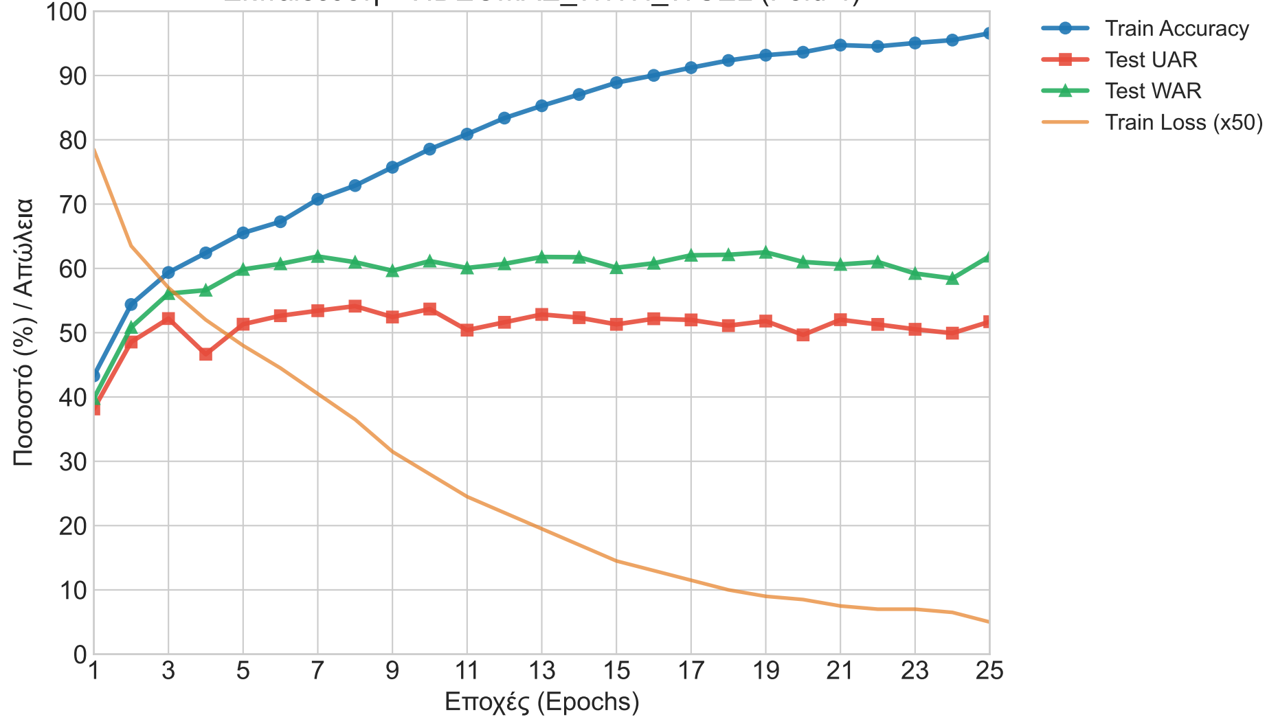
Εκπαίδευση - VIDEOMAE_WITH_WCEL (Fold 4)
