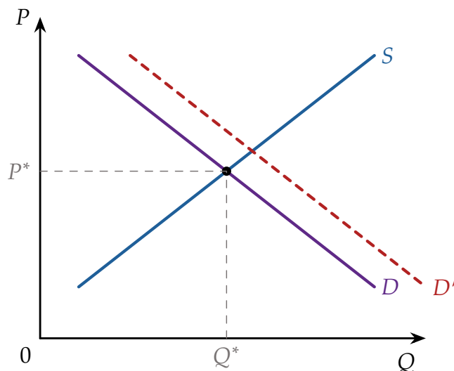
Gráfico 1 – Equilibrio y desplazamiento de la demanda
