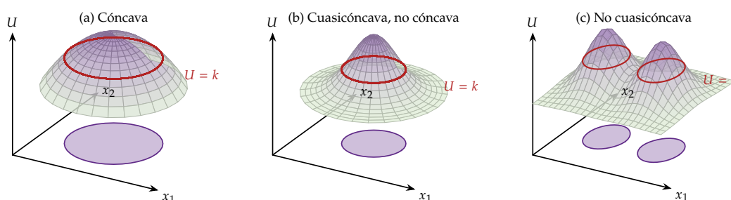
Gráfico 4 – Cuasiconcavidad: función cóncava, función cuasicóncava y función que no es cuasicóncava
