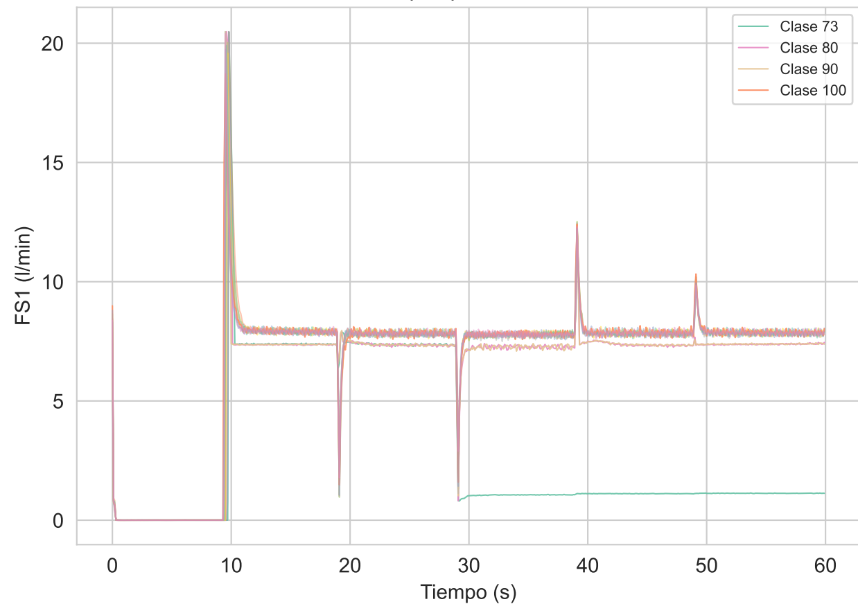
Caudal 1 (FS1) vs Válvula — H2
