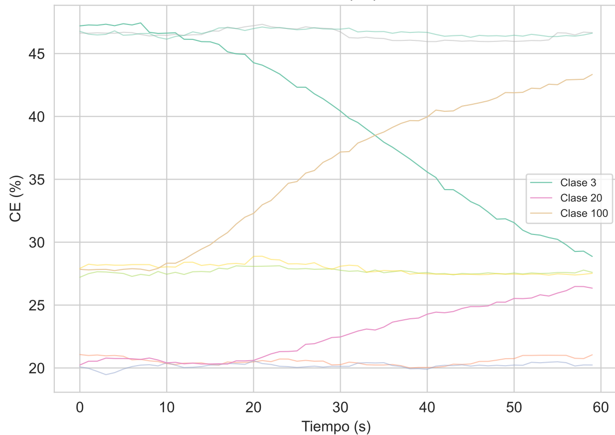
Eficiencia Enfriamiento (CE) vs Cooler — H1
