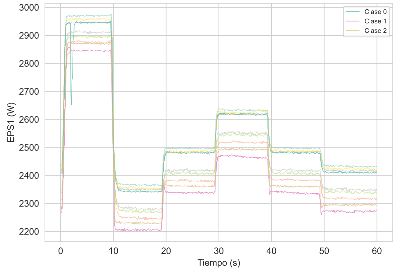
Potencia Motor (EPS1) vs Bomba — H3
